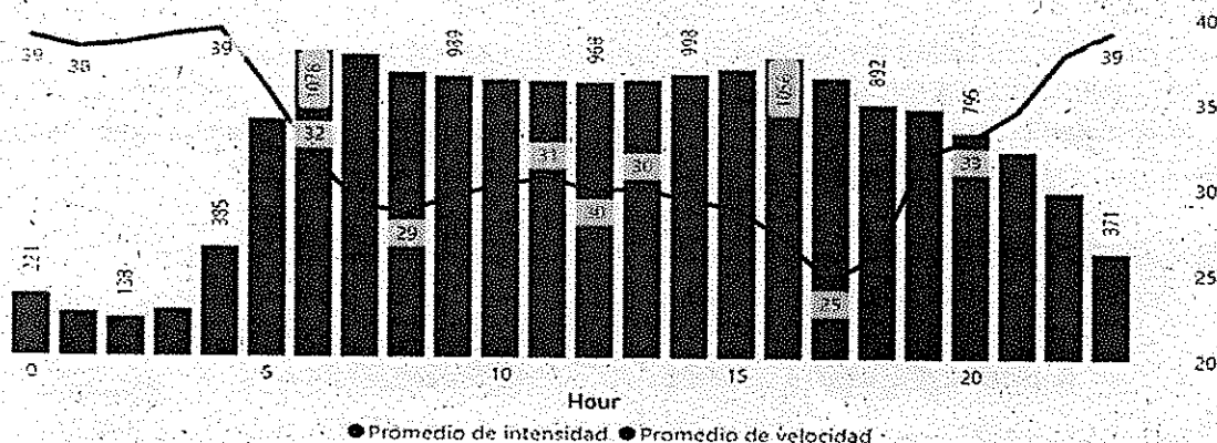
Figura 6. Intensidad y velocidad vehicular promedio por hora en día típico en vías exentas. Semestre 2 de 2024
