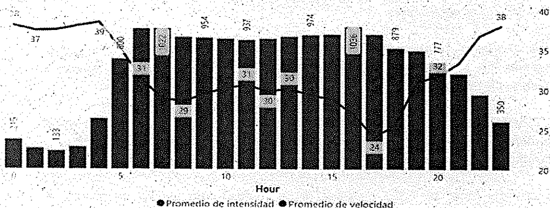
Figura 5. Intensidad y velocidad vehicular promedio por hora en día típico en vías exentas. Semestre 1 de 2024
