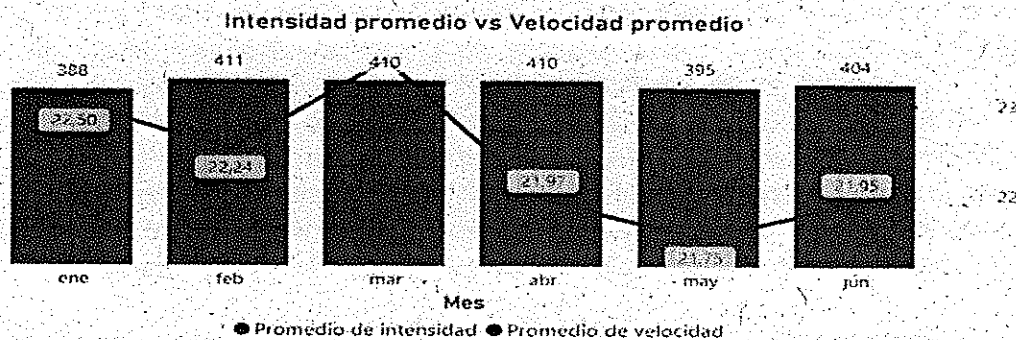
Figura 1. Intensidad y velocidad vehicular horaria promedio por mes para día típico en vías con la medida de PyP.
