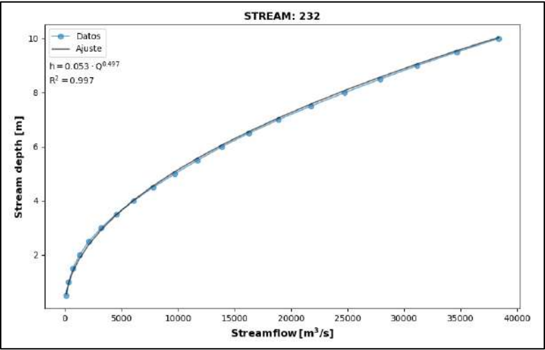
Figura 78 Curva de calibración nivel-caudal en el tramo de descarga de la quebrada La Corralita. Fuente: Estudio básico de amenazas Caldas (2023)
