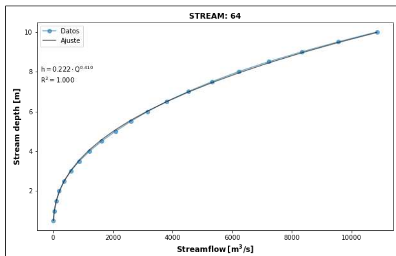
Figura 18. Curva de calibración nivel-caudal en el tramo de descarga de la quebrada La Miel.
