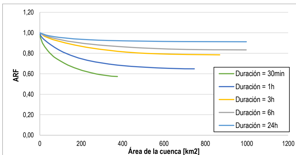
Figura 9. Curvas de factor de reducción de la lluvia por área
