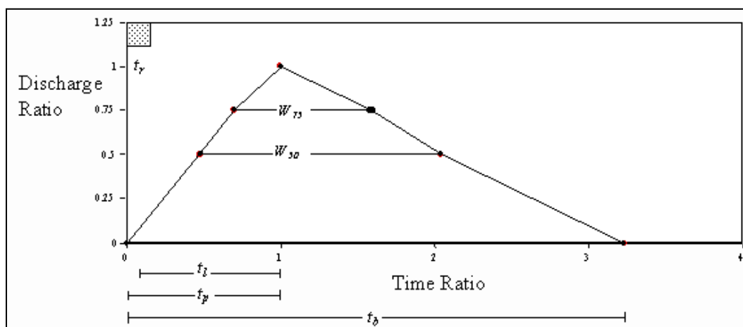
Figura 11. Hidrograma unitario sintético de Snyder Fuente: (Ramírez, 2000).
