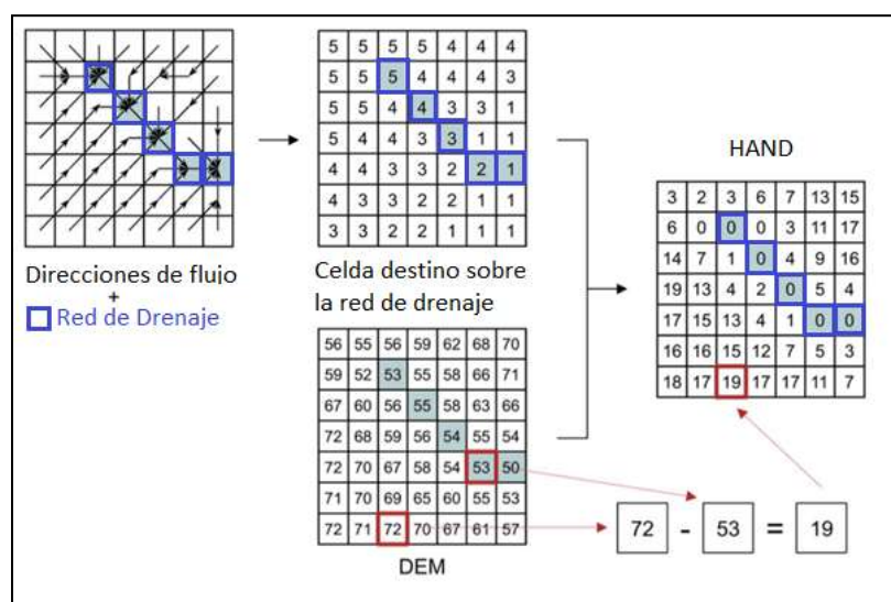
Figura 16. Esquematización del mapa de inundaciones asociado al DEM y niveles máximos.
