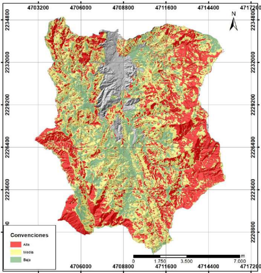
Figura 87. Amenaza de movimientos en masa de tipo rotacional en suelo rural en escenarios: (c) Escenario 3; (d) Escenario 4. Fuente: Estudio básico de amenazas Caldas (2023)
