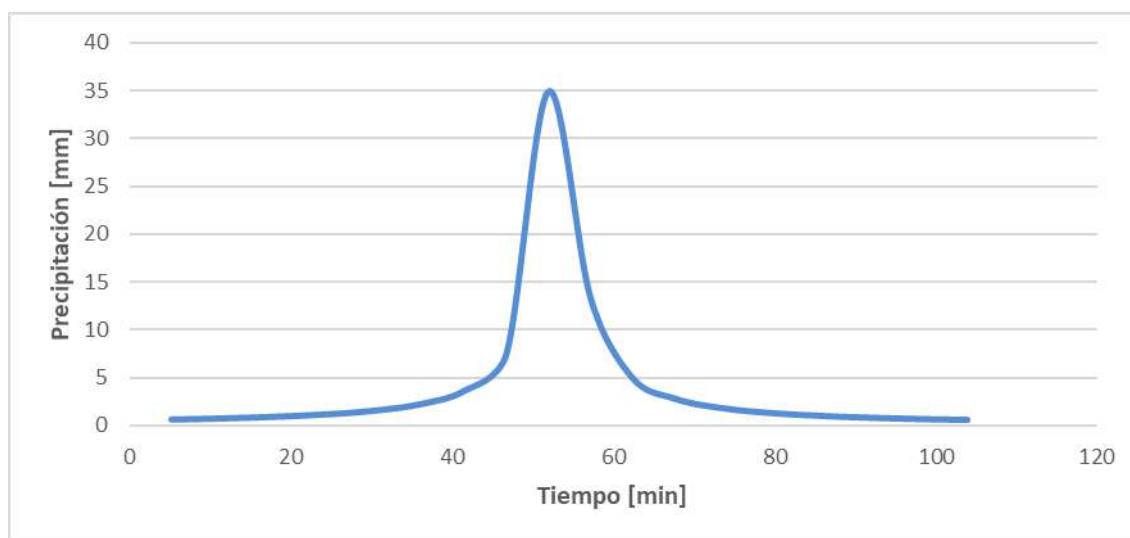
Figura 64. Distribución temporal de la precipitación con un período de retorno de 100 años en la Q. La Valeria.
