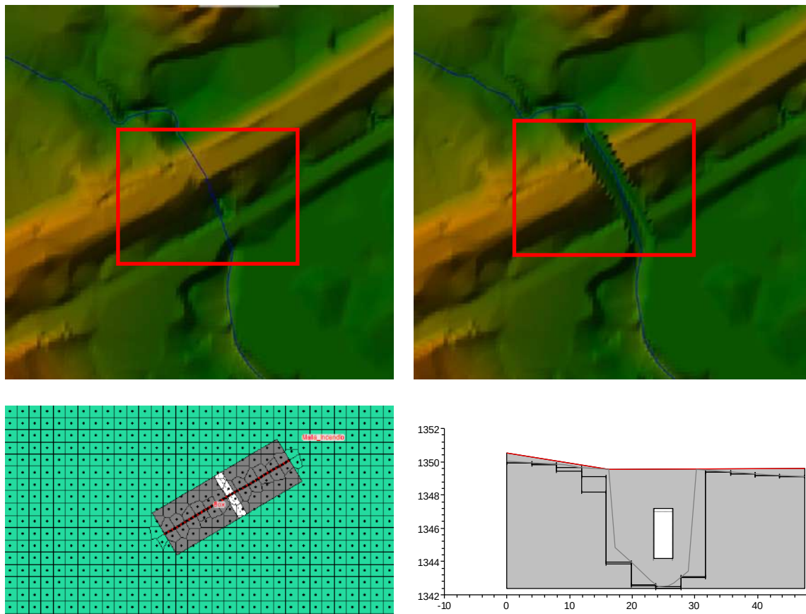
Figura 76 Ajuste del modelo digital de elevación para la implantación de una estructura hidráulica en la quebrada La Miel. Fuente: Estudio básico de amenazas Caldas (2023)
