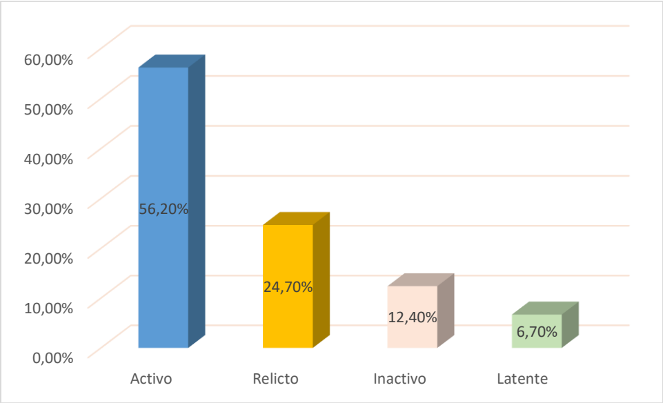
Gráfico 16. Estado de los procesos morfodinámicos identificados en suelo urbano y de expansión. Fuente: Estudio básico de amenazas Caldas (2023)
