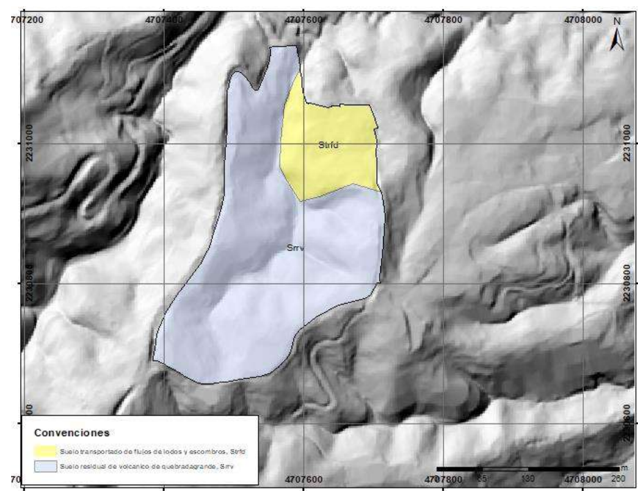
Figura 119. Mapa de formaciones superficiales del centro poblado La Chuscala Fuente: Estudio básico de amenazas Caldas (2023)
