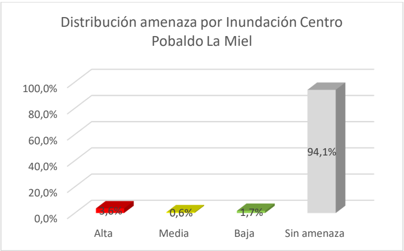
Gráfico 46. Distribución de amenaza por inundación en el centro poblado La Miel. Fuente: Estudio básico de amenazas Caldas (2023)
