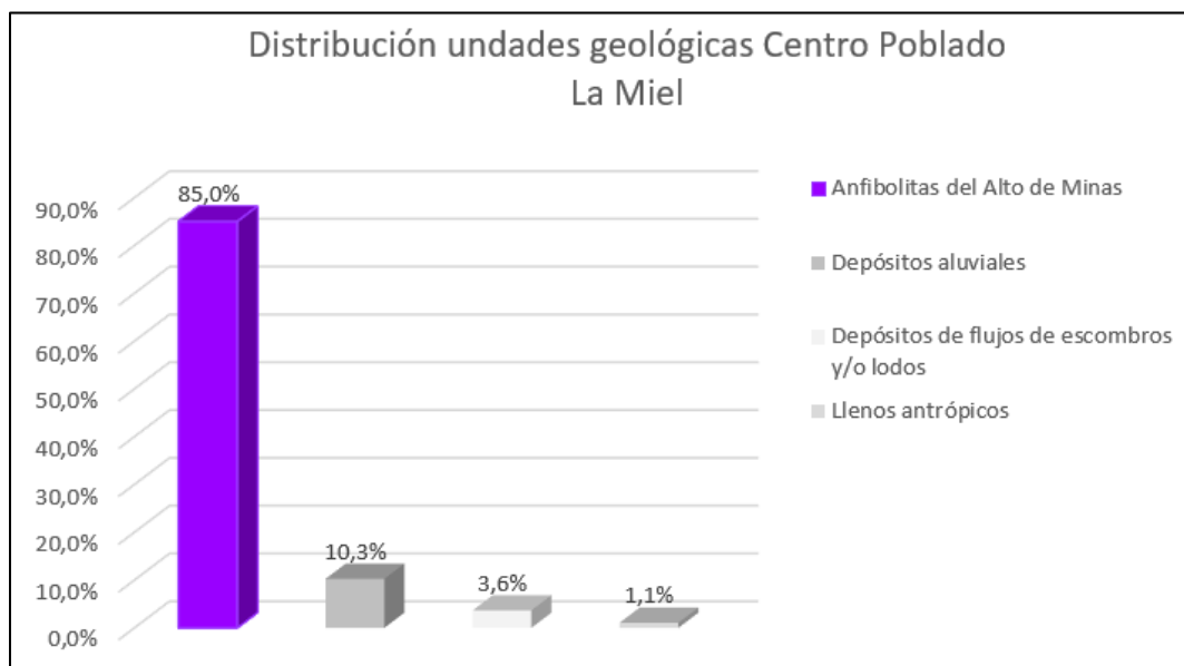
Gráfico 42. Distribución de unidades geológicas en el centro poblado La Miel.
