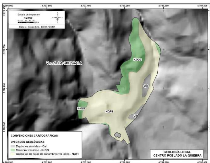
Figura 146. Mapa de unidades geológicas del centro poblado La Quebra.
