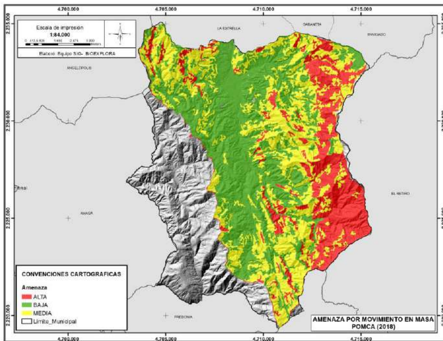
Figura 99. Mapa de amenaza por movimiento en masa, POMCA (2018). Fuente: Tomado y modificado del POMCA (2018)
