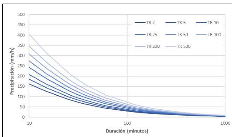
Figura 8. Curvas de IDF en la estación Caldas en condiciones futuras (cambio climático).
