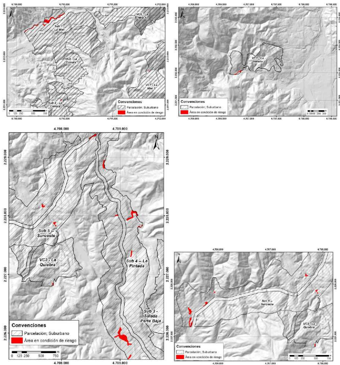
Figura 194. Áreas con condición de riesgo por inundación en suelos suburbanos y de parcelación Fuente: Estudio básico de amenazas del municipio de Caldas 2023
