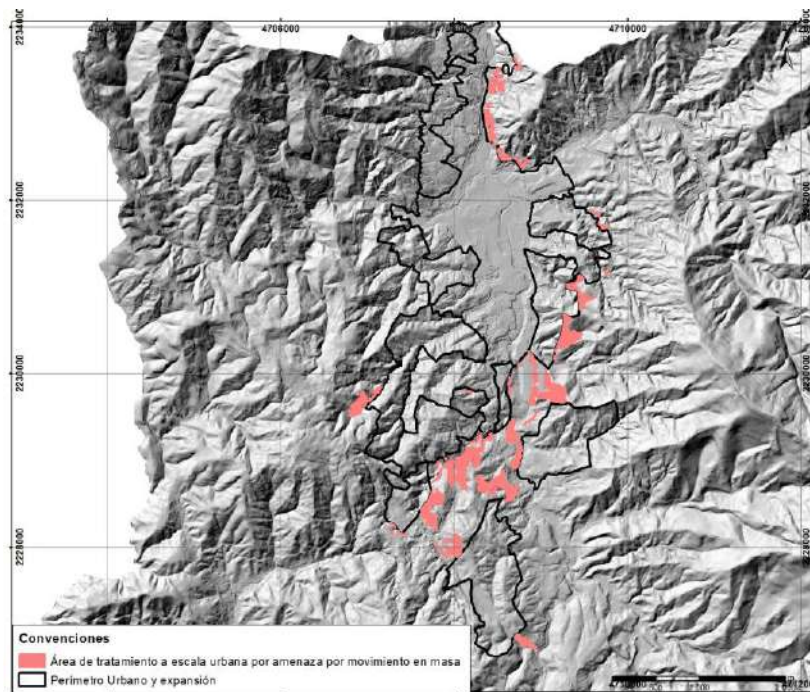
Figura 183. Mapa de áreas de población limítrofes al perímetro urbano con tratamiento a escala urbana por amenaza por movimiento en masa.
