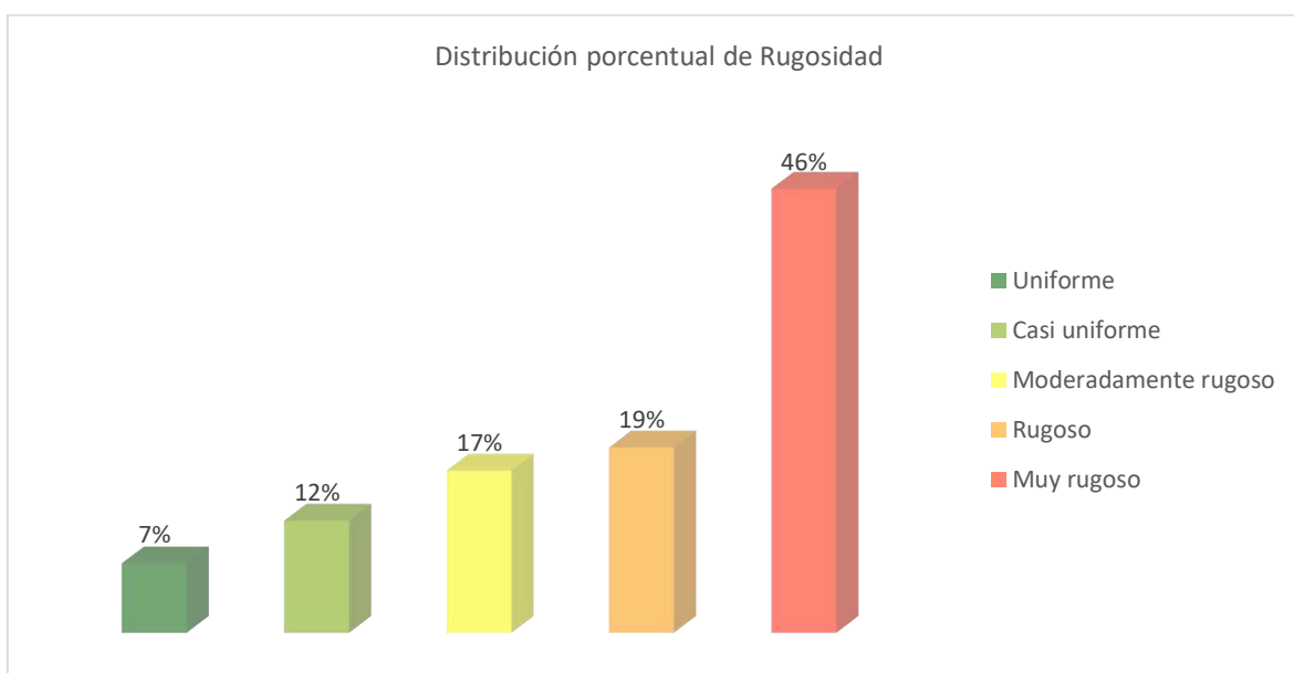
Gráfico 9. Distribución porcentual de la rugosidad del terreno. Fuente: Estudios básicos de amenaza Caldas (2023)
