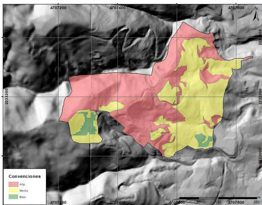
Figura 116. Mapa de amenaza por movimientos en masa para el centro poblado La Aguacatala.
