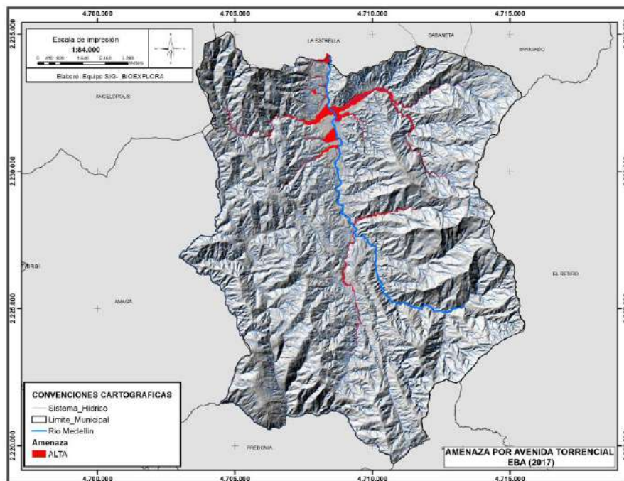
Figura 105. Mapa de amenaza por avenida torrencial, (UNAL & AMVA, 2018)
