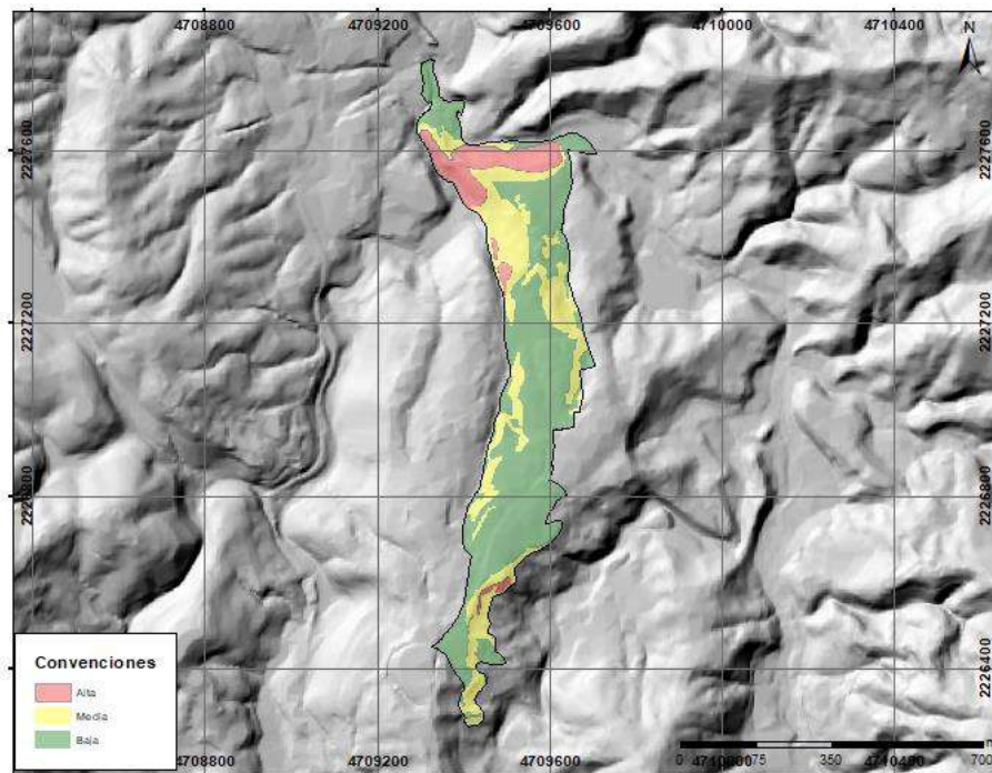
Figura 169. Mapa de amenaza por movimiento en masa para el centro poblado La Salada parte baja. Fuente: Estudio básico de amenazas Caldas (2023)
