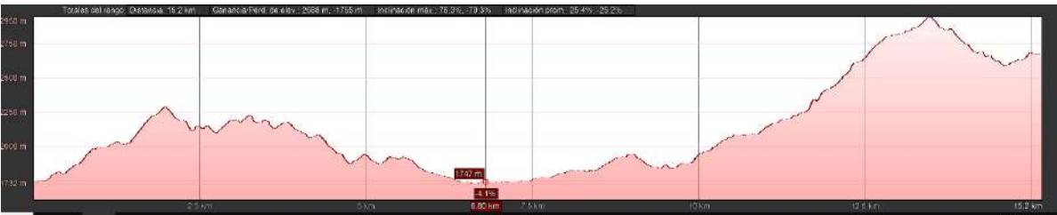
Gráfico 1. Perfil del territorio municipal, occidente a oriente, a la altura de primavera, La línea marca la divisoria de aguas, Aburrá Cauca.
