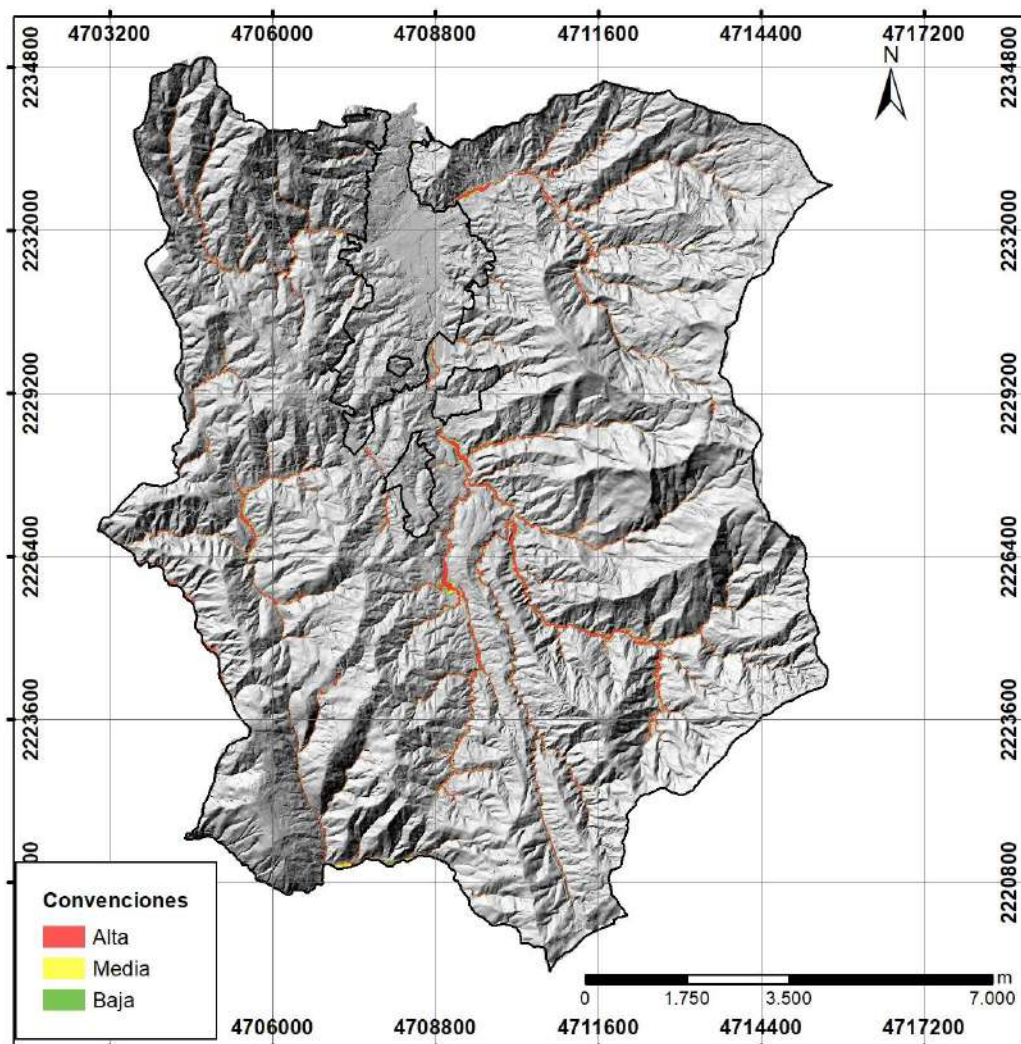
Figura 91. Mapa de amenaza por inundación para suelo rural del municipio de Caldas. Fuente: Estudio básico de amenazas Caldas (2023)
