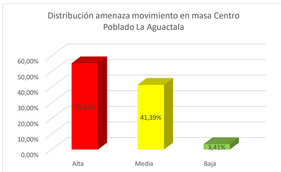
Gráfico 27. Distribución porcentual de amenaza por Movimiento en masa en el centro poblado La Aguacatala.
