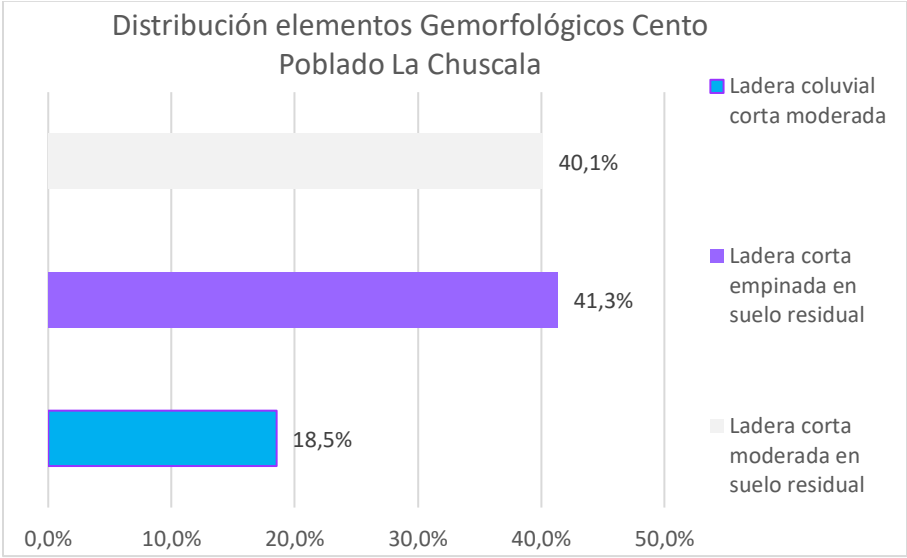
Gráfico 30. Distribución de unidades geomorfológicas en el centro poblado La Chuscala. Fuente: Estudio básico de amenazas Caldas (2023)
