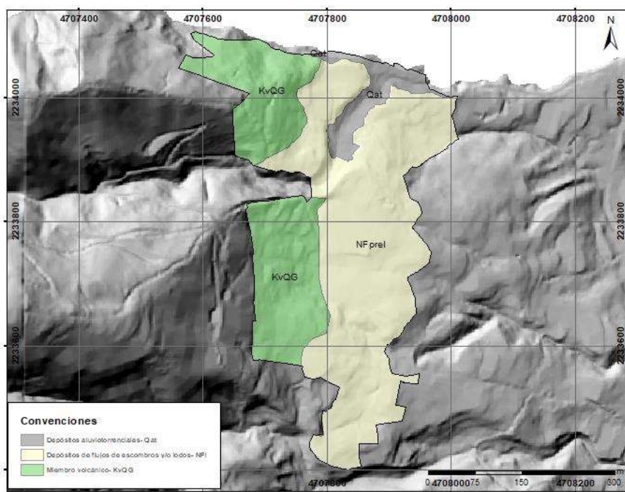
Figura 154. Mapa de unidades geológicas del centro poblado La Raya.
