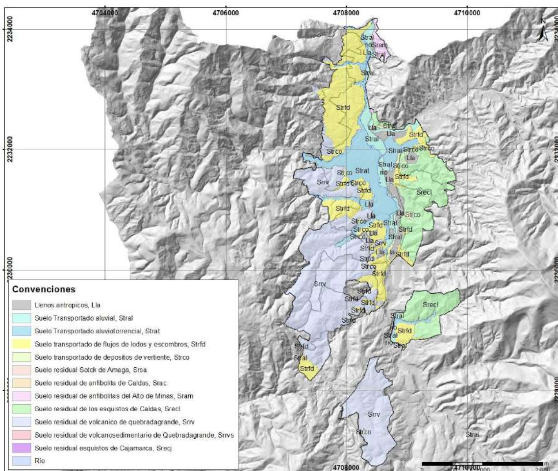
Figura 40. Mapa de las formaciones superficiales presentes en el suelo urbano y de expansión del municipio de Caldas.
