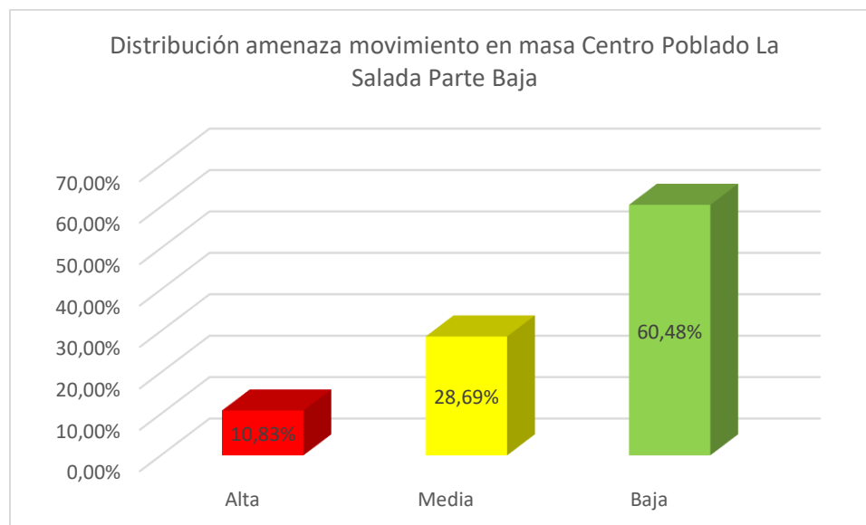
Gráfico 61. Distribución porcentual de amenaza por Movimiento en masa en el centro poblado La Salada parte baja. Fuente: Estudio básico de amenazas Caldas (2023)
