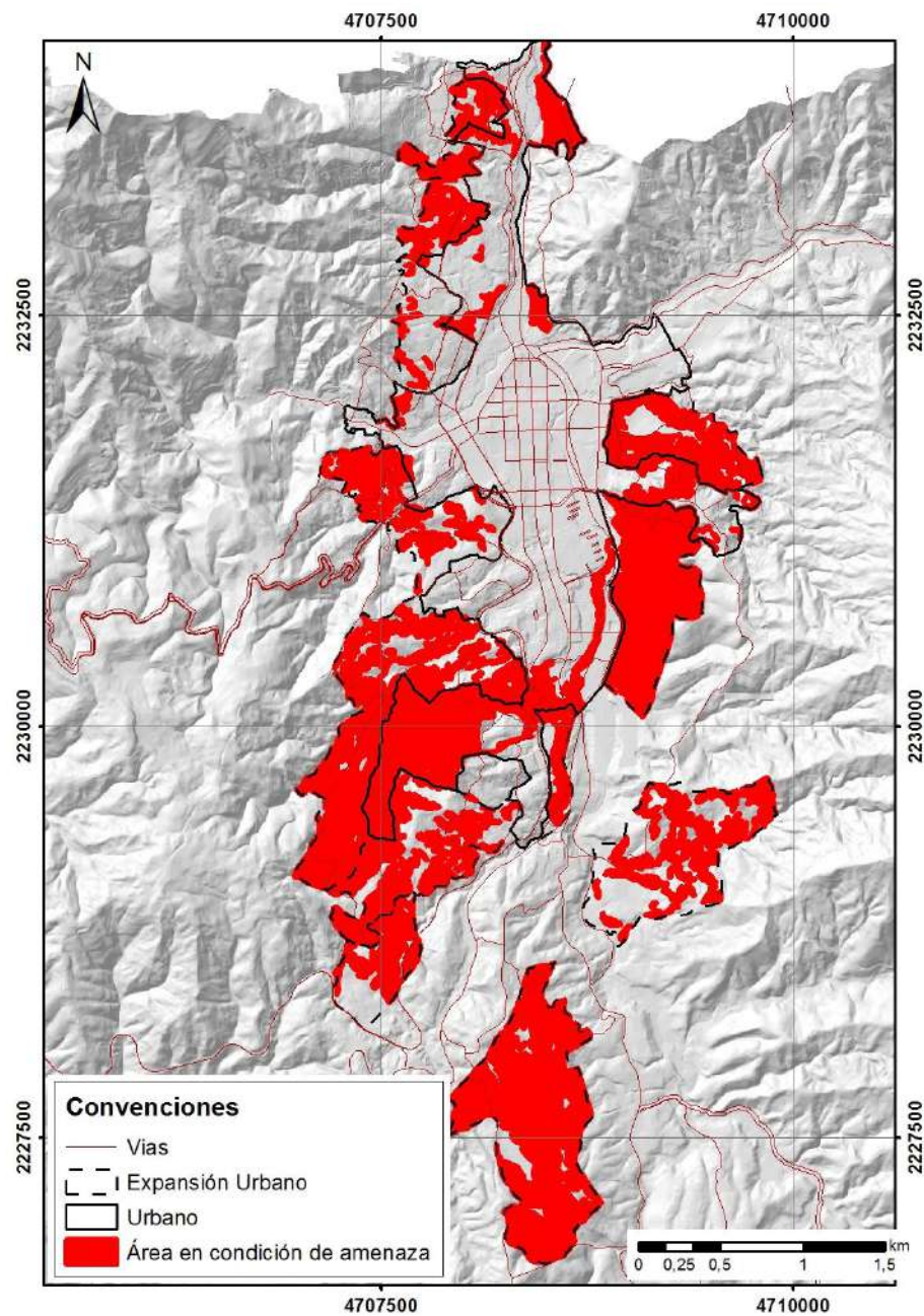
Figura 204. Áreas con condición de amenaza por movimientos en masa en suelo urbano y expansión.
