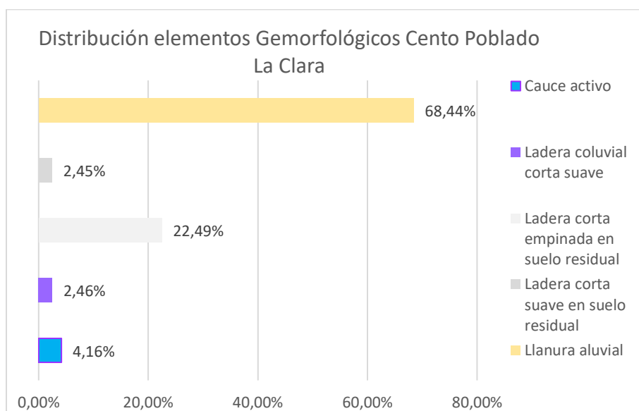
Gráfico 34. Distribución de unidades geomorfológicas en el centro poblado La Clara.
