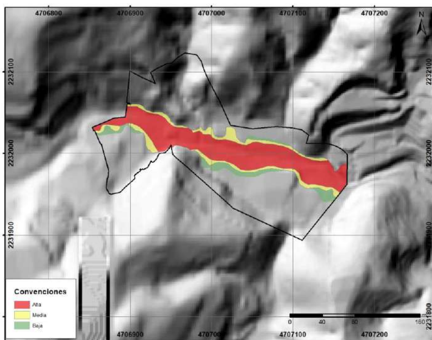
Figura 177. Mapa de amenaza por inundación para el centro poblado La Valeria.
