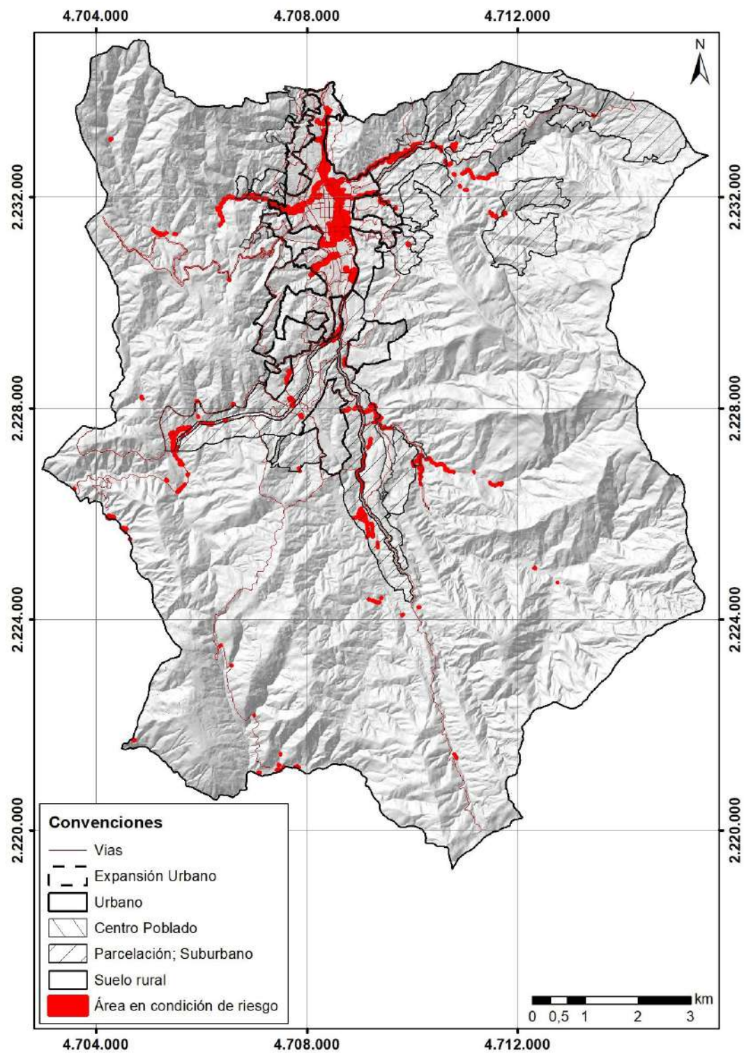
Figura 197. Áreas con condición de riesgo por avenida torrencial para el municipio de Caldas. Fuente: Estudio básico de amenazas del municipio de Caldas 2023
