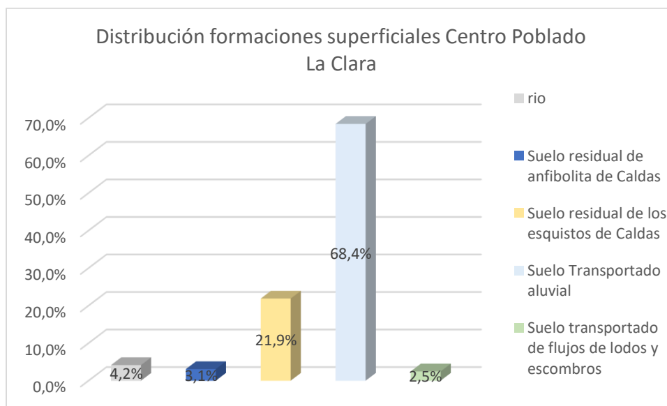
Gráfico 33. Distribución de formaciones superficiales en el centro poblado La Clara Fuente: Estudio básico de amenazas Caldas (2023)
