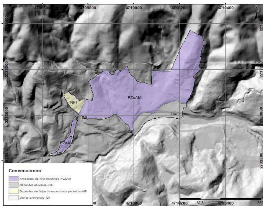
Figura 138. Mapa de unidades geológicas del centro poblado La Miel. Fuente: Estudio básico de amenazas Caldas (2023)
