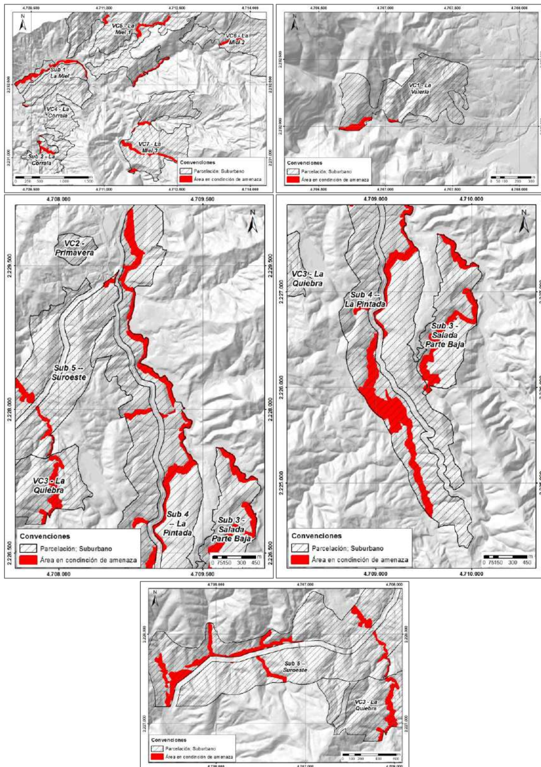
Figura 213. Áreas con condición de amenaza por avenida torrencial en suelo suburbano y parcelación. Fuente: Estudio básico de amenazas del municipio de Caldas 2023
