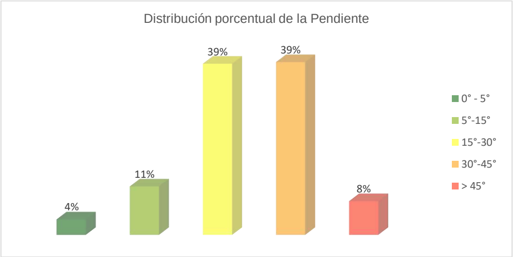
Gráfico 8. Distribución porcentual de la pendiente en el municipio de Caldas. Fuente: Estudios básicos de amenaza Caldas (2023)
