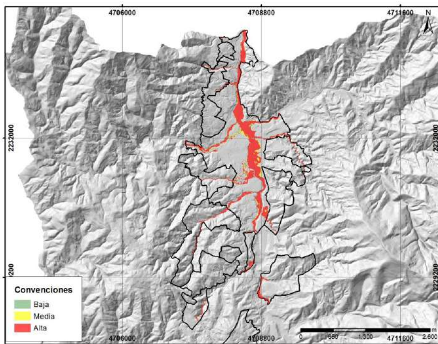
Figura 92. Clasificación amenaza por avenida torrencial acorde a modelación hidráulica
