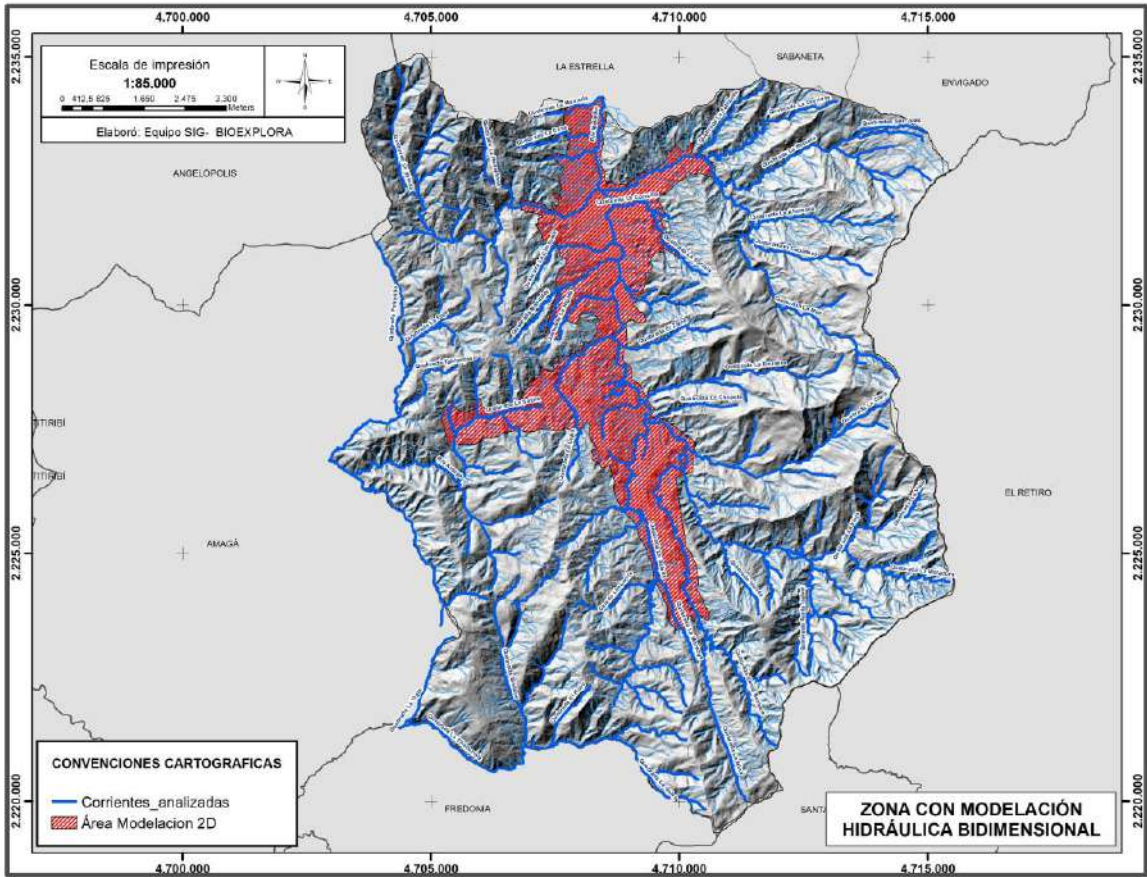
Figura 70. Zonas con modelación hidráulica bidimensional. Fuente: Estudio básico de amenazas Caldas (2023)
