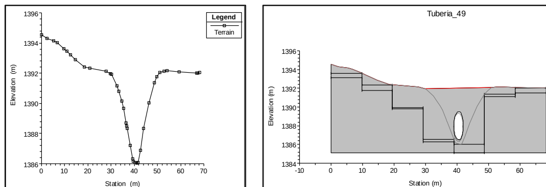
Figura 74 Implantación de estructura hidráulica en el modelo digita del terreno de la quebrada La Miel. Fuente: Estudio básico de amenazas Caldas (2023)
