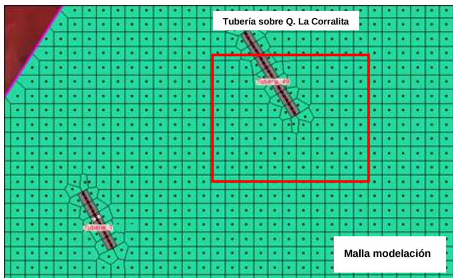
Figura 75. Implantación de la estructura en la malla de modelado 2D. Fuente: Estudio básico de amenazas Caldas (2023)
