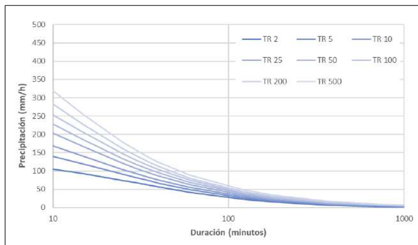
Figura 7. Curvas de IDF en la estación Caldas en condiciones actuales. Fuente: (AMVA, 2018)
