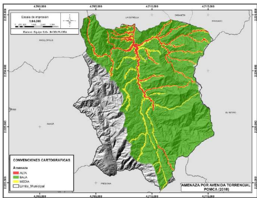
Figura 106. Mapa de amenaza por avenida torrencial, POMCA (2018).
