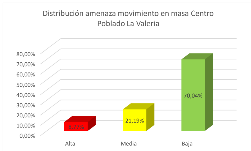
Gráfico 65. Distribución porcentual de amenaza por Movimiento en masa en el centro poblado La Valeria. Fuente: Estudio básico de amenazas Caldas (2023)
