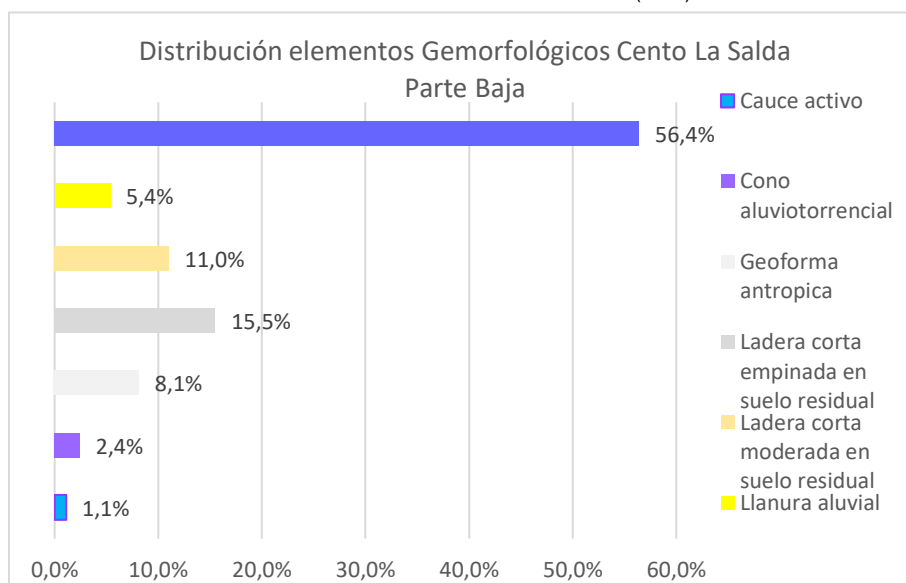
Gráfico 60. Distribución de unidades geomorfológicas en el centro poblado La Salada parte baja.
