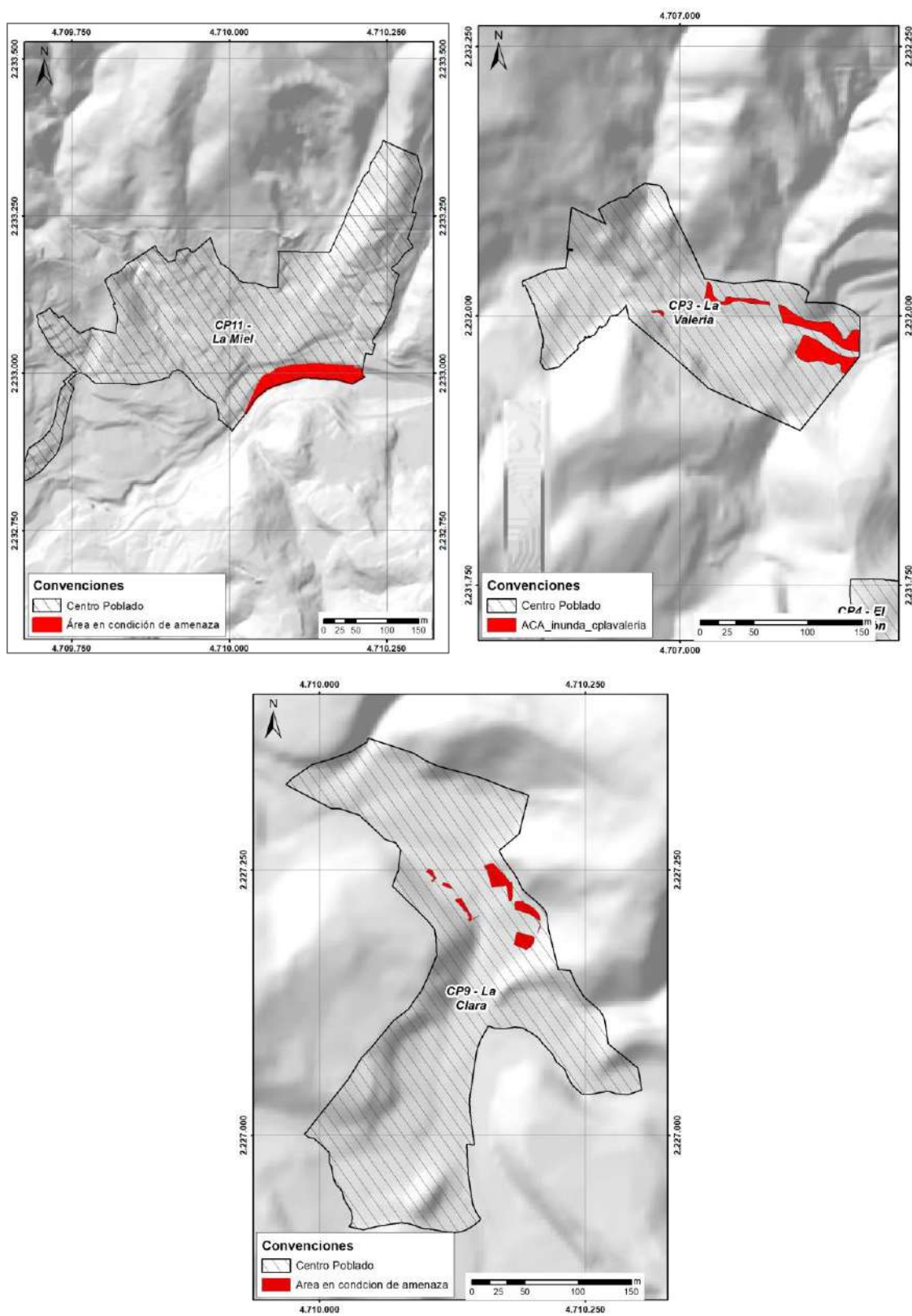
Figura 210. Áreas con condición de amenaza por inundación en centros poblados. Fuente: Estudio básico de amenazas del municipio de Caldas 2023.
