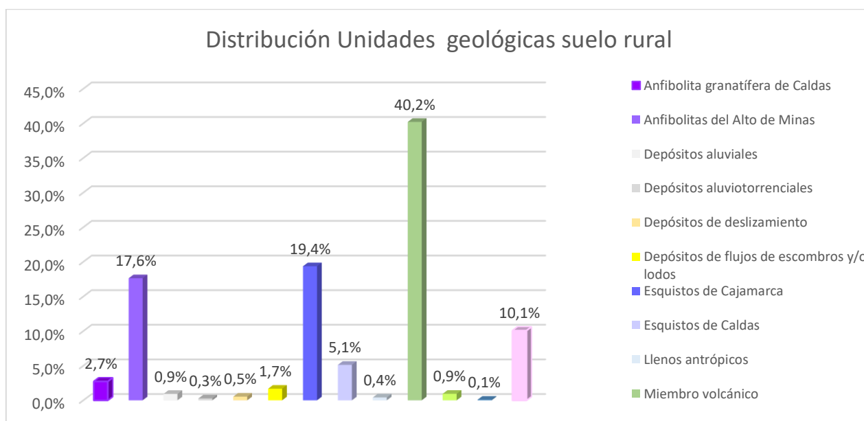
Gráfico 12. Distribución de unidades geológicas en suelo rural del municipio de Caldas.
