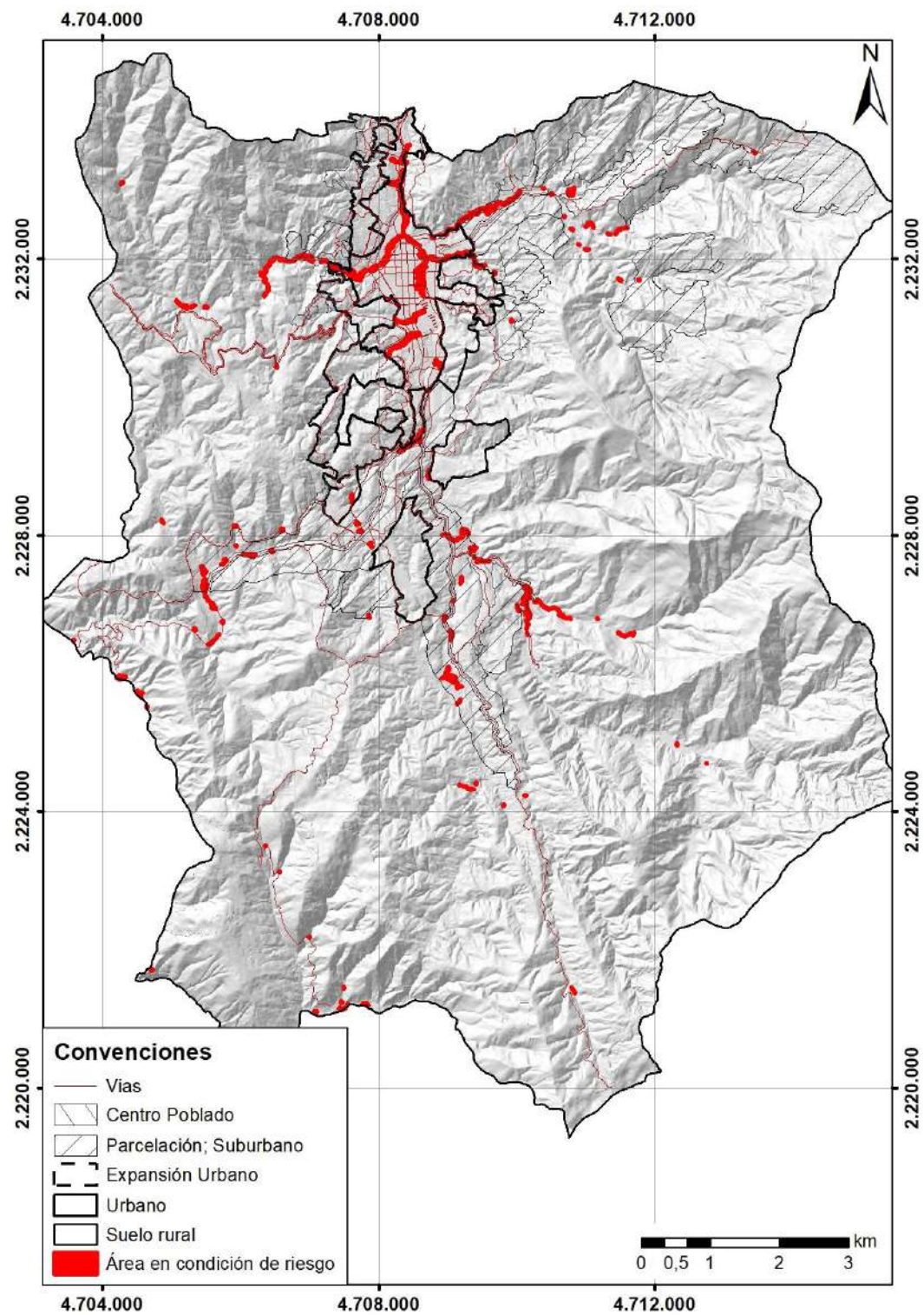
Figura 192. Áreas con condición de riesgo por inundación para el municipio de Caldas. Fuente: Estudio básico de amenazas del municipio de Caldas 2023
