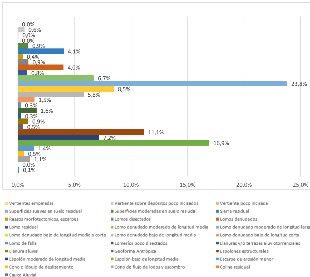
Gráfico 15. Distribución de unidades geomorfológicas en suelo rural del municipio de Caldas.
