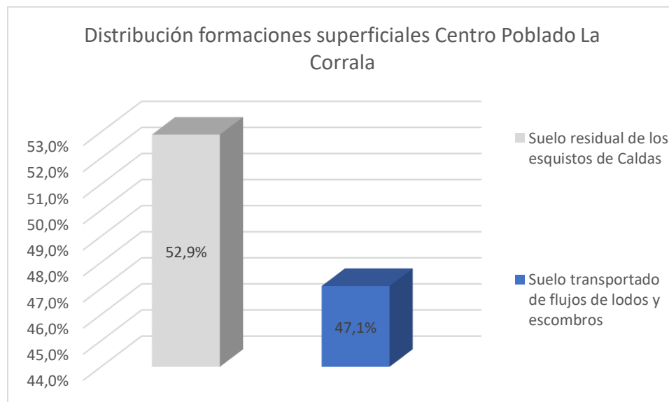
Gráfico 39. Distribución de formaciones superficiales en el centro poblado La Corrala Fuente: Estudio básico de amenazas Caldas (2023)
