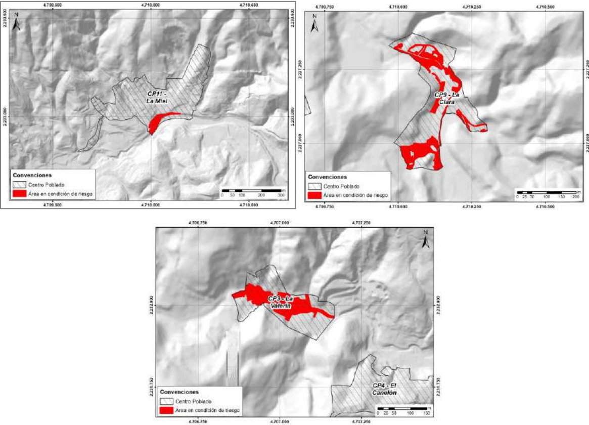
Figura 200. Áreas con condición de riesgo por avenida torrencial en centros poblados. Fuente: Estudio básico de amenazas del municipio de Caldas 2023
