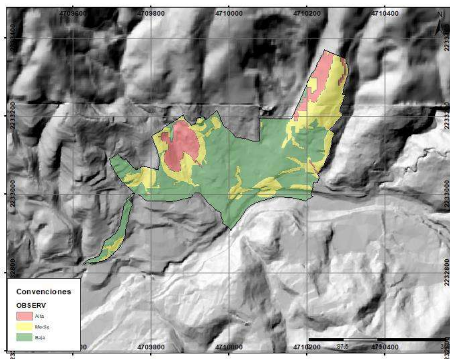
Figura 143. Mapa de amenaza por movimiento en masa para el centro poblado La Miel.
