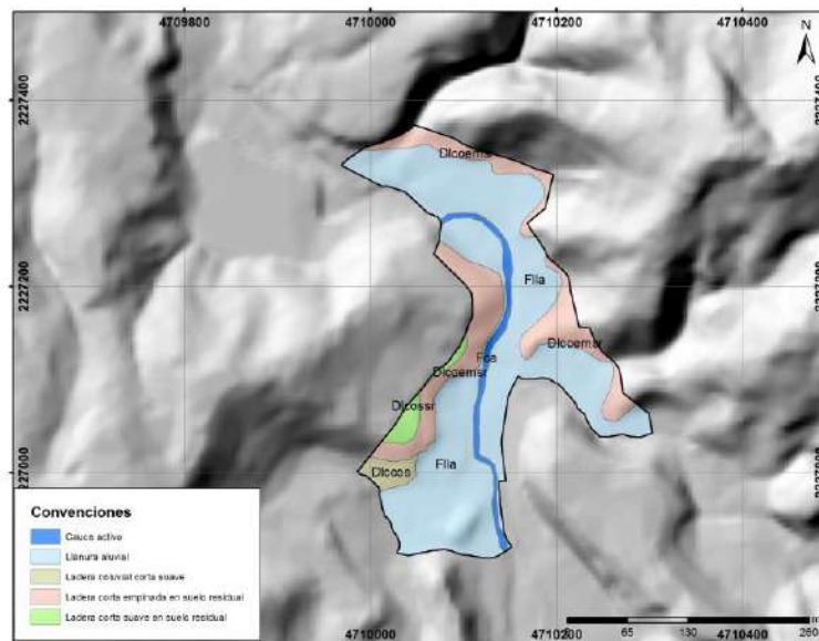
Figura 128. Mapa de unidades geomorfológicas del centro poblado La Clara.
