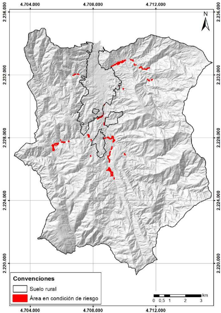
Figura 201. Áreas con condición de riesgo por avenida torrencial en suelo rural. Fuente: Estudio básico de amenazas del municipio de Caldas 2023
