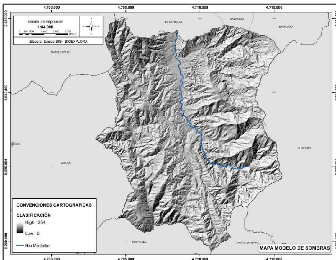
Figura 20. Modelo de sombras del municipio de Caldas. Fuente: Estudios básicos de amenaza Caldas (2023)
