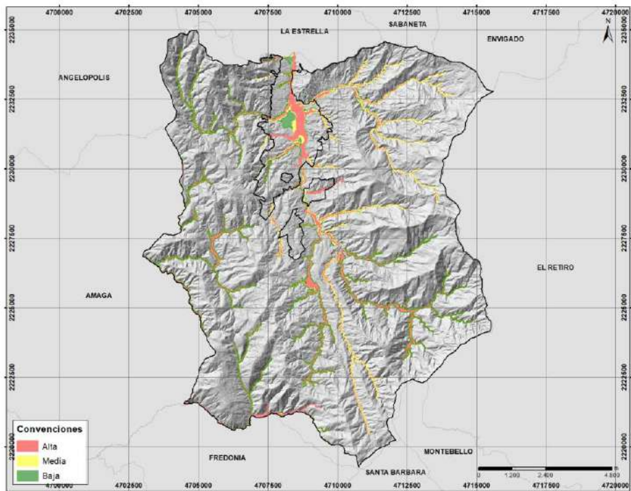
Figura 107. Mapa de amenaza por avenida torrencial del presente estudio.
