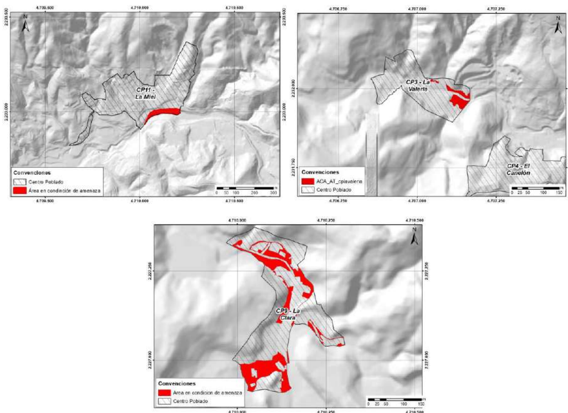
Figura 214. Áreas con condición de amenaza por avenida torrencial en centros poblados
