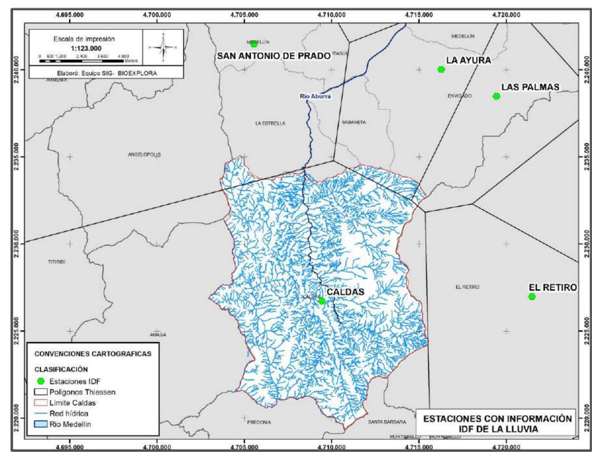
Figura 6. Estaciones con información de IDF de la lluvia Fuente: Estudios básicos de amenaza Caldas (2023)
