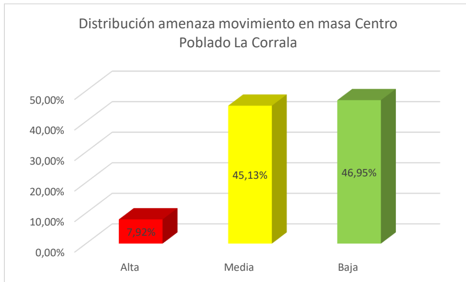
Gráfico 41. Distribución porcentual de amenaza por Movimiento en masa en el centro poblado La Corrala. Fuente: Estudio básico de amenazas Caldas (2023)
