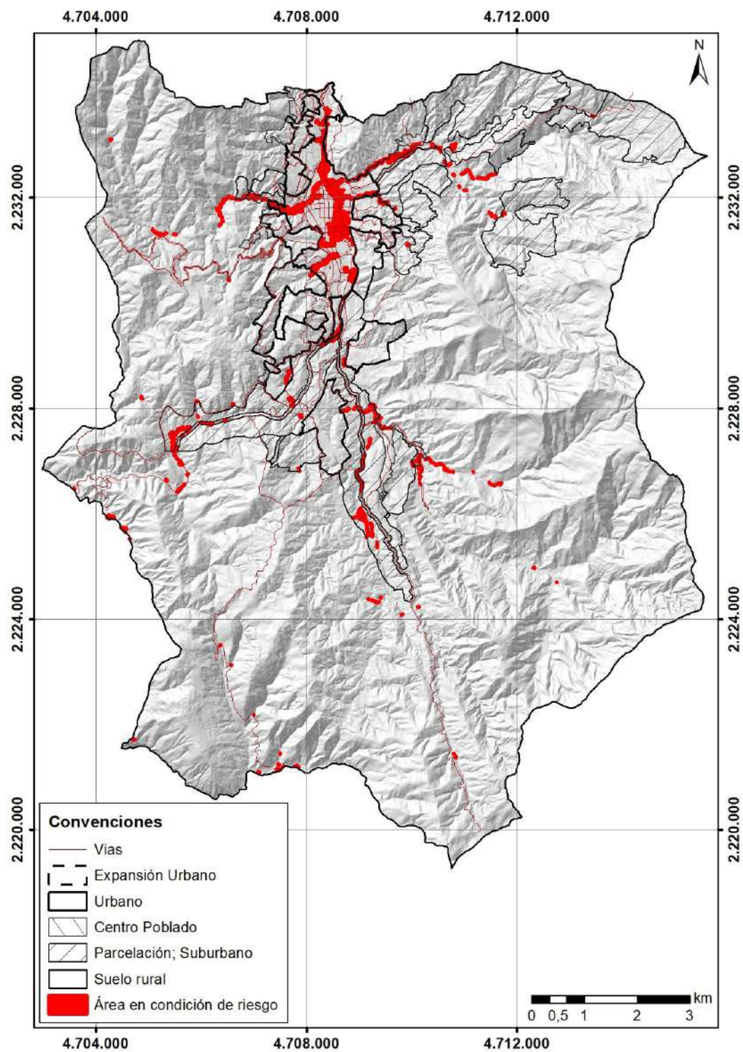
Figura 211. Áreas con condición de amenaza por avenida torrencial para el municipio de Caldas. Fuente: Estudio básico de amenazas del municipio de Caldas 2023.
