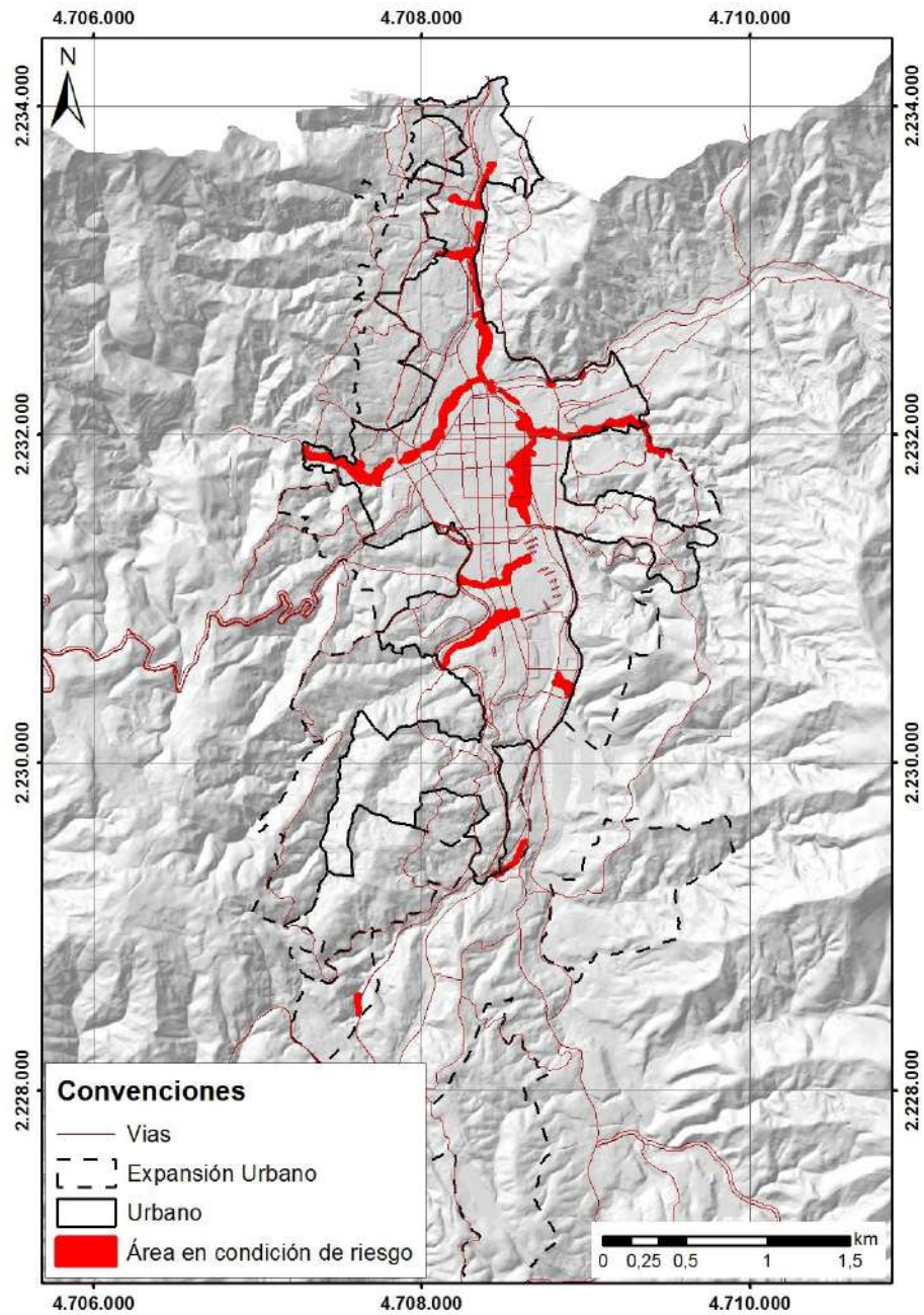
Figura 193. Áreas con condición de riesgo por inundación en suelo urbano y expansión. Fuente: Estudio básico de amenazas del municipio de Caldas 2023
