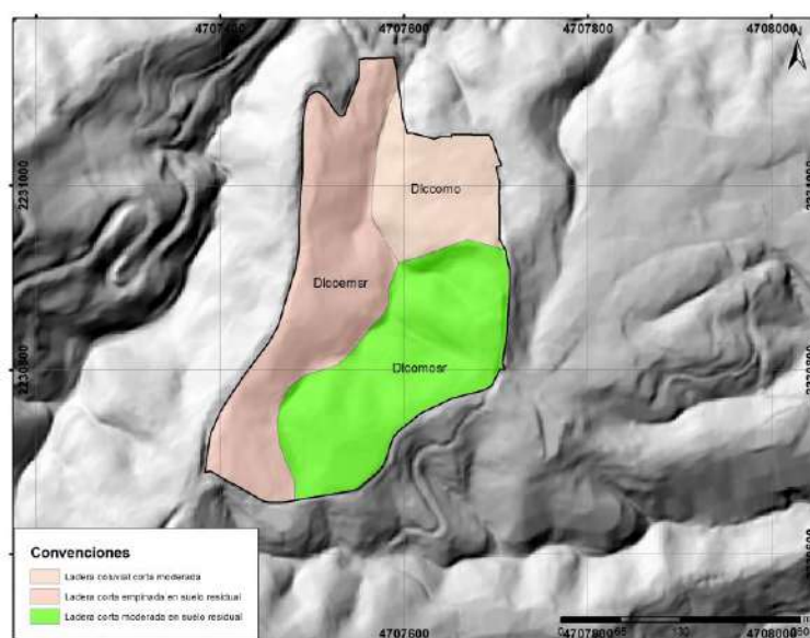
Figura 120. Mapa de unidades geomorfológicas del centro poblado La Chuscala. Fuente: Estudio básico de amenazas Caldas (2023)
