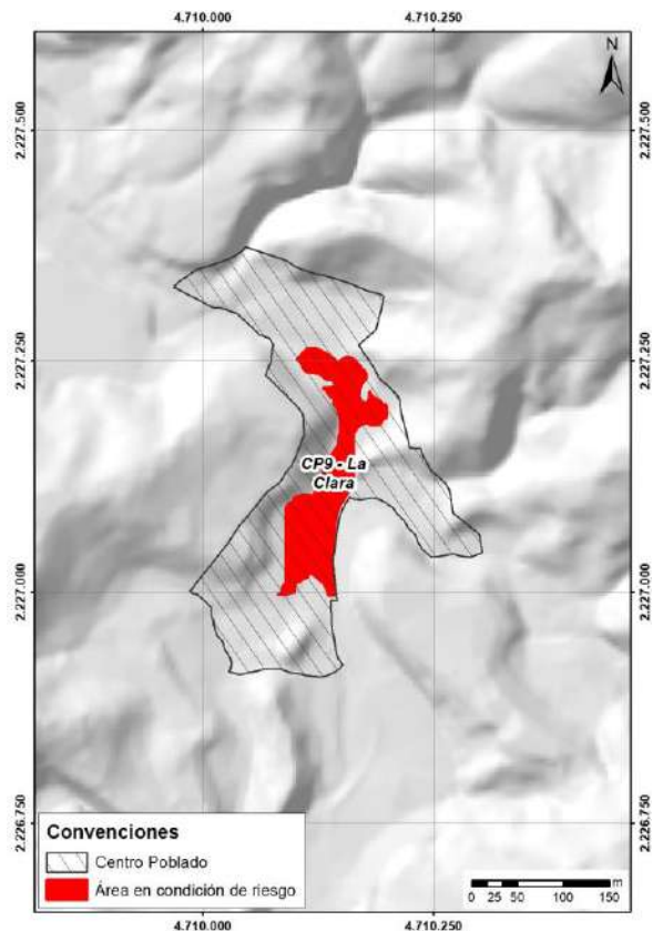
Figura 195. Áreas con condición de riesgo por inundación para centros poblados. Fuente: Estudio básico de amenazas del municipio de Caldas 2023
