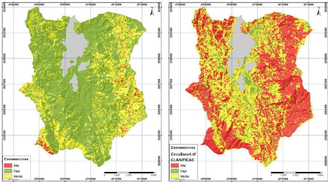
Figura 87. Amenaza de movimientos en masa de tipo rotacional en suelo rural en escenarios: (c) Escenario 3; (d) Escenario 4. Fuente: Estudio básico de amenazas Caldas (2023)
