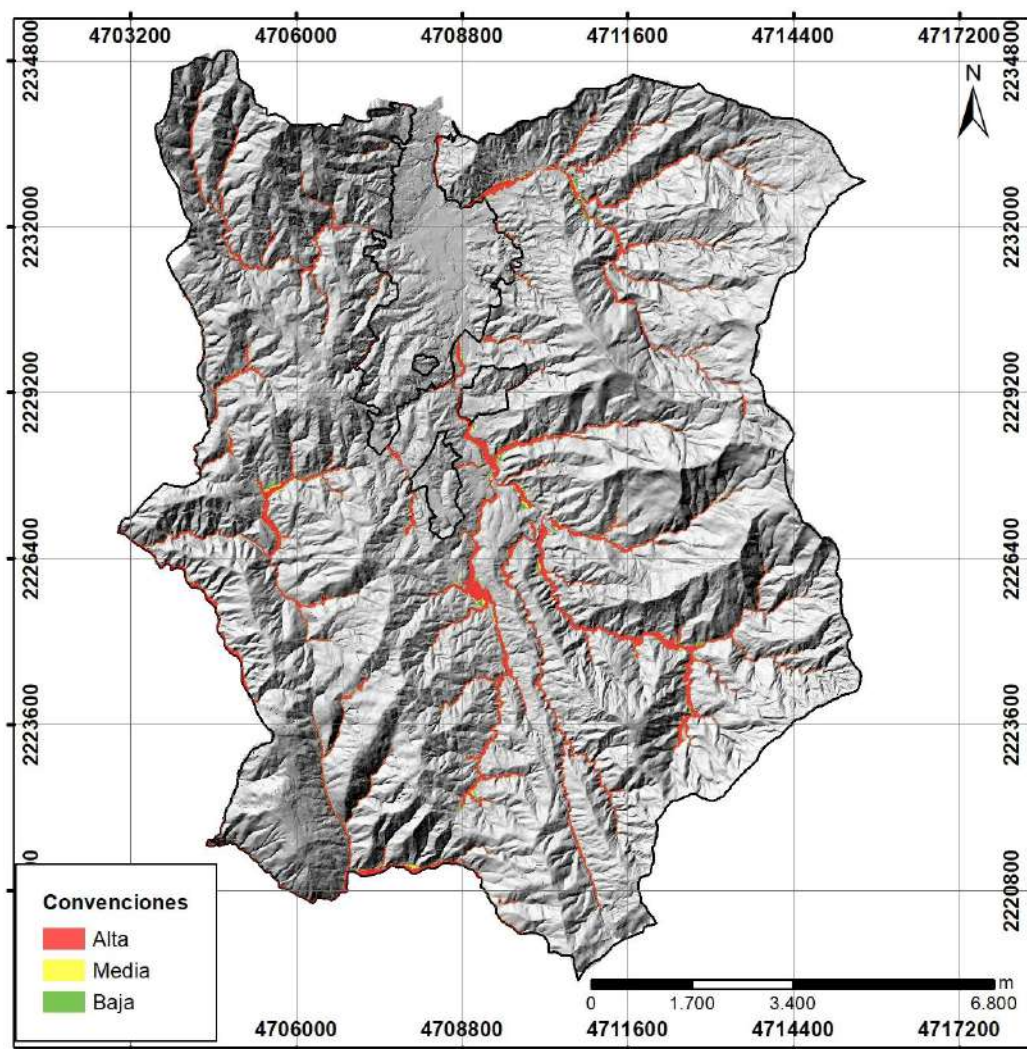
Figura 96. Mapa de amenaza por avenida torrencial para suelo rural del municipio de Caldas. Fuente: Estudio básico de amenazas Caldas (2023)
