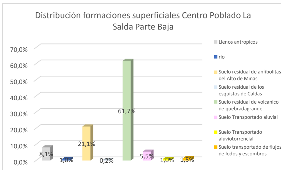
Gráfico 59. Distribución de formaciones superficiales en el centro poblado La Salada Parte Baja Fuente: Estudio básico de amenazas Caldas (2023)
