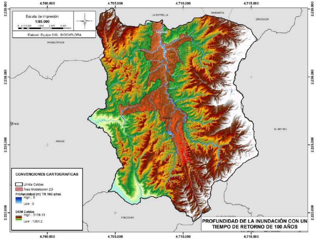
Figura 79 Profundidad de la inundación con un TR de 100 años, metodología HAND – Zona Rural y Urbana 1 Fuente: Estudio básico de amenazas Caldas (2023)
