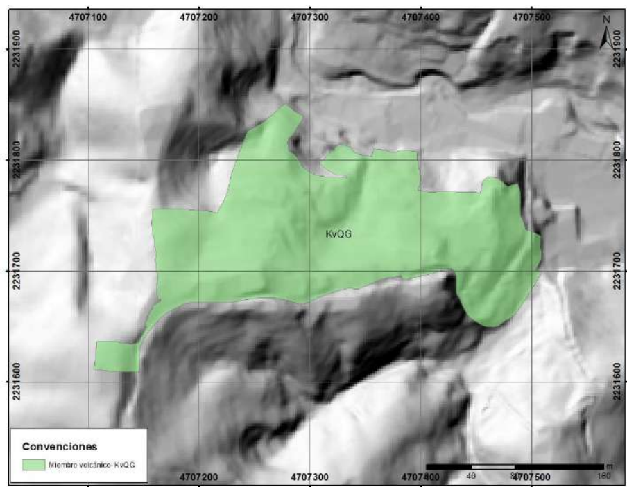
Figura 108. Mapa de unidades geológicas del centro poblado El Canelón Fuente: Estudio básico de amenazas Caldas (2023)
