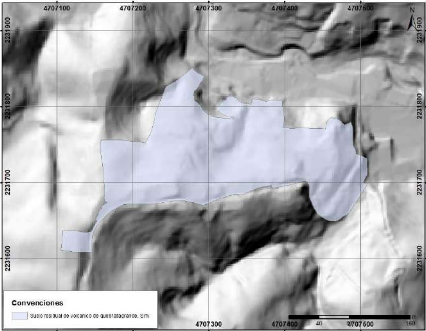
Figura 109. Mapa de formaciones superficiales del centro poblado El Canelón Fuente: Estudio básico de amenazas Caldas (2023)
