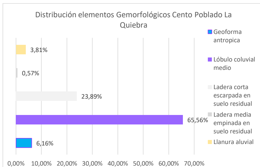
Gráfico 50. Distribución de unidades geomorfológicas en el centro poblado La Quiebra. Fuente: Estudio básico de amenazas Caldas (2023)
