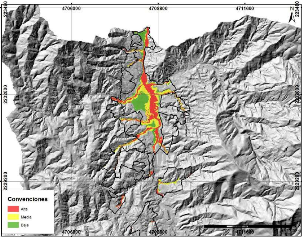
Figura 94. Mapa de amenaza por avenida torrencial para suelo urbano y de expansión del municipio de Caldas. Fuente: Estudio básico de amenazas Caldas (2023)
