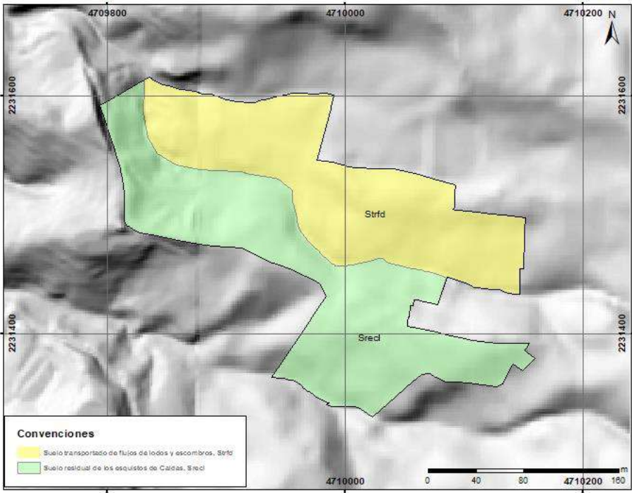
Figura 135. Mapa de formaciones superficiales del centro poblado La Corrala Fuente: Estudio básico de amenazas Caldas (2023)
