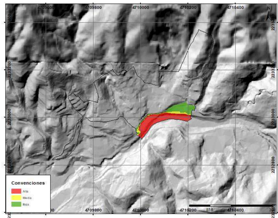
Figura 145. Mapa de amenaza por avenida torrencial para el centro poblado La Miel. Fuente: Estudio básico de amenazas Caldas (2023)
