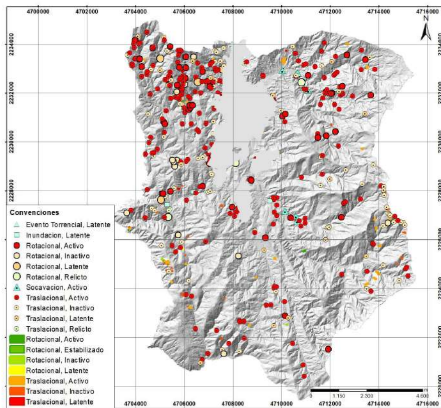
Figura 53. Mapa de procesos morfodinámicos en suelo rural. Fuente: Estudio básico de amenazas Caldas (2023)
