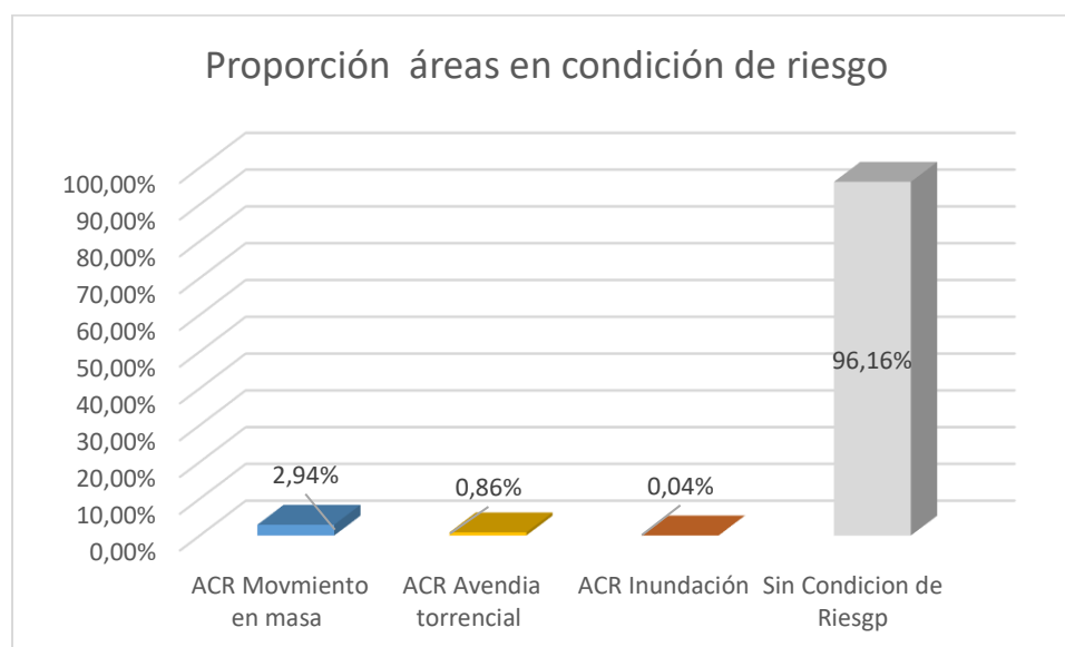
Figura 186. Proporción de áreas con condición de riesgo respecto al municipio de Caldas.
