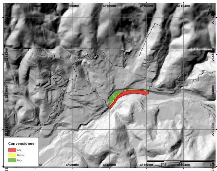
Figura 144. Mapa de amenaza por inundación para el centro poblado La Miel. Fuente: Estudio básico de amenazas Caldas (2023)
