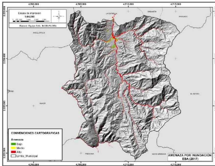
Figura 102. Mapa de amenaza por inundación, (UNAL &amp; AMVA, 2018)
