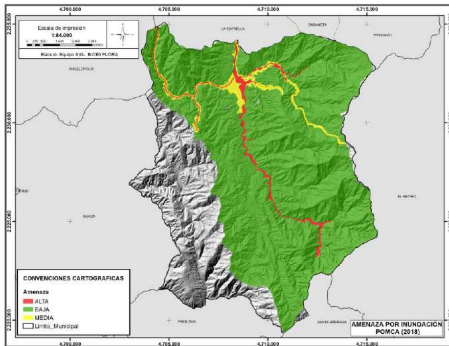
Figura 103. Mapa de amenaza por inundación, POMCA (2018).
