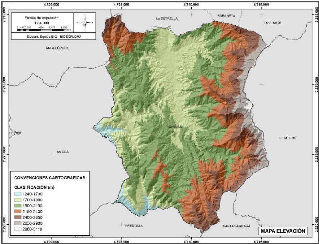
Figura 19. Modelo de elevación digital (DEM) para el municipio de Caldas. Fuente: Estudios básicos de amenaza Caldas (2023)
