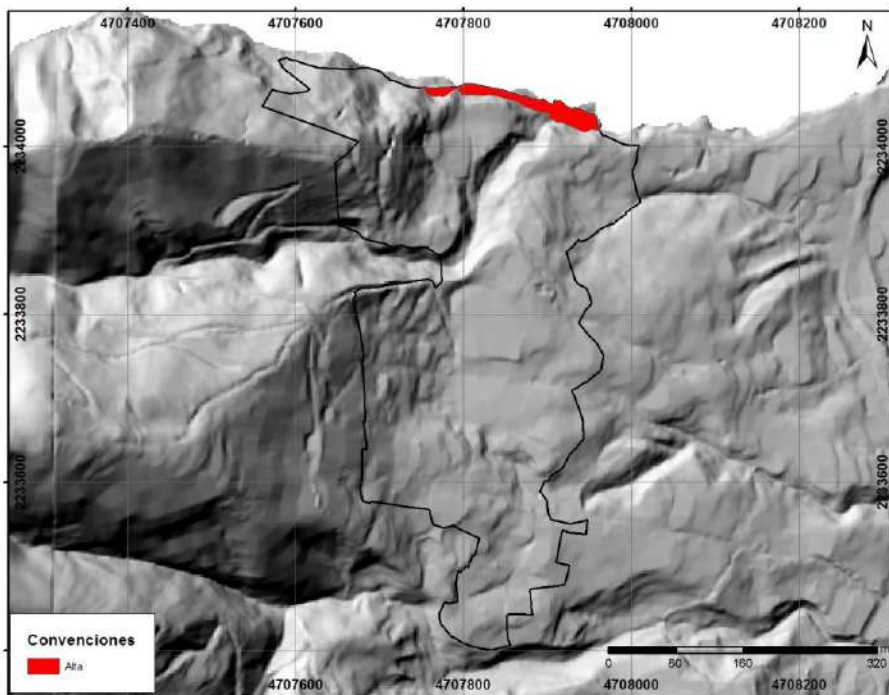
Figura 163. Mapa de amenaza por avenida torrencial para el centro La Raya.
