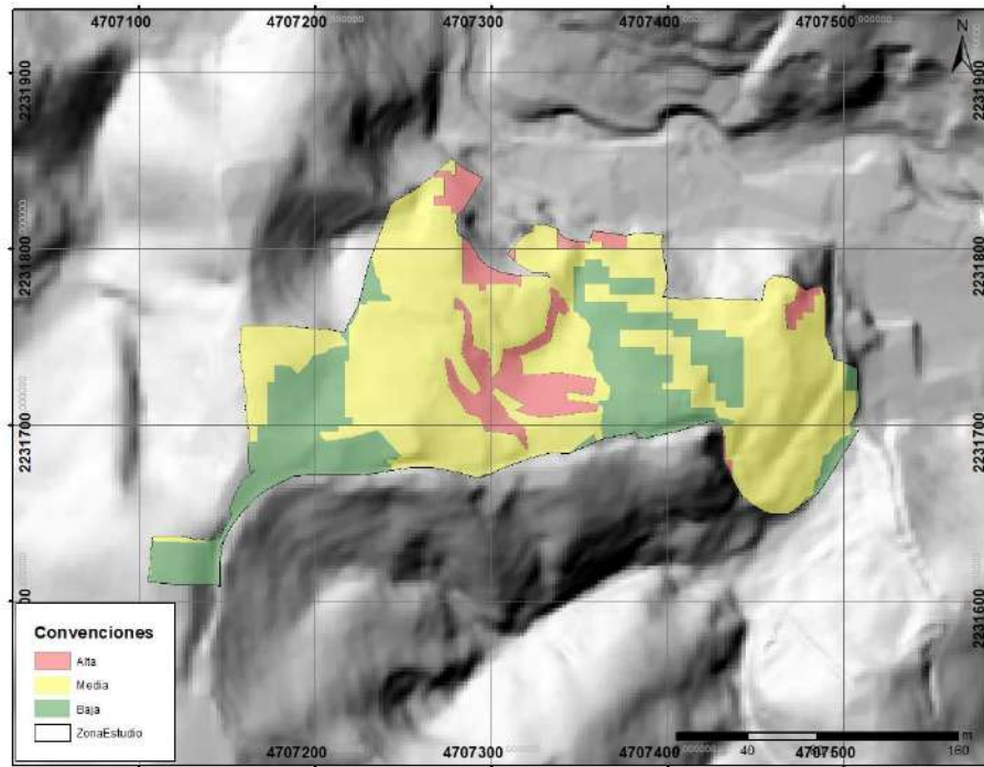
Figura 111. Mapa de amenaza por movimientos en masa para el centro poblado El Canelón Fuente: Estudio básico de amenazas Caldas (2023)
