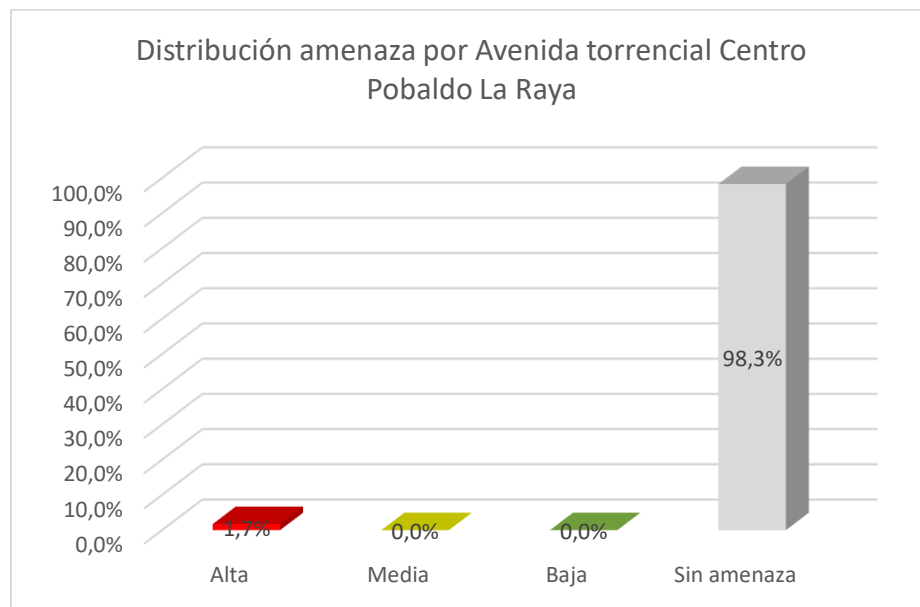
Gráfico 57. Distribución porcentual de amenaza por avenida torrencial en el centro poblado La Raya. Fuente: Estudio básico de amenazas Caldas (2023)
