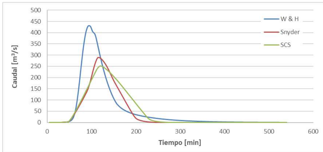
Figura 69. Hidrógrafa de respuesta estimada por las diferentes metodologías en la quebrada La Miel ante la ocurrencia del evento de precipitación asociado a un periodo de retorno de 200 años.
