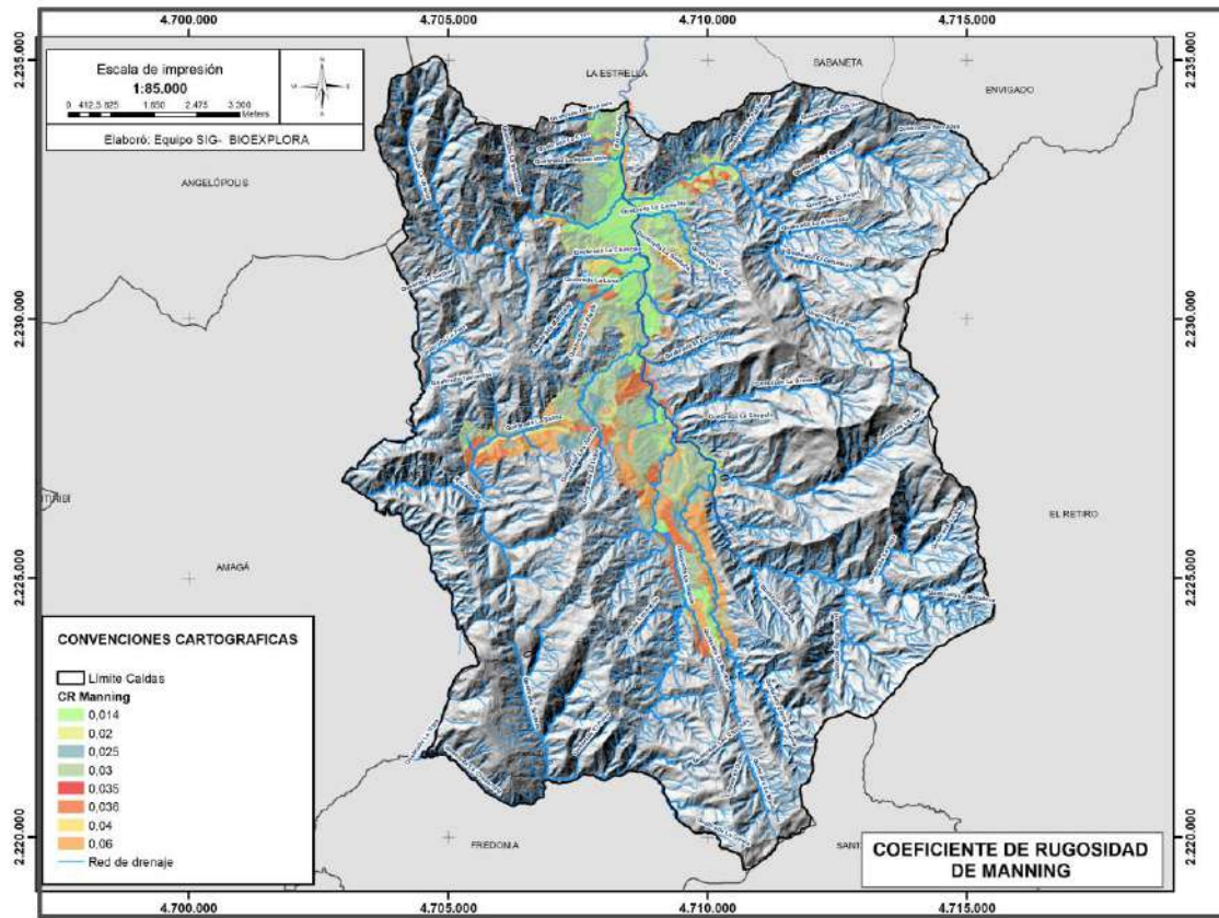
Figura 77. Coeficiente de rugosidad de Maning Fuente: Estudio básico de amenazas Caldas (2023)
