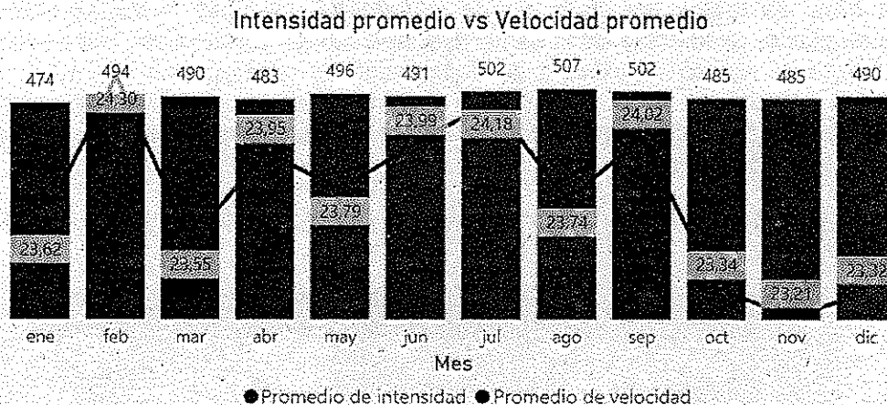
Figura 1. Intensidad y velocidad vehicular horaria promedio por mes para día típico. Año 2023.
