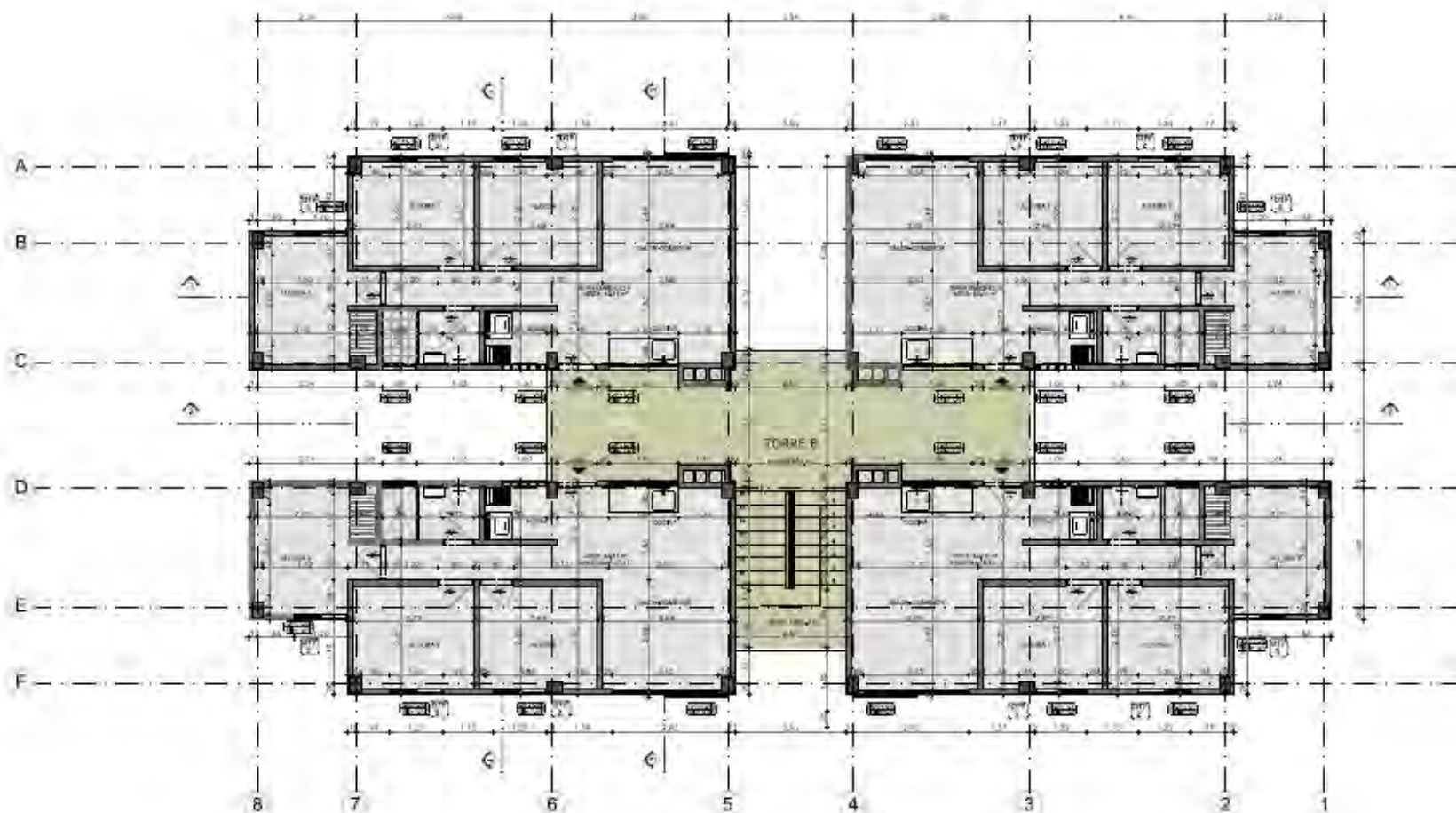
PLANTA TIPO TORRES 1-4 y 8-11 ESC 1:50
